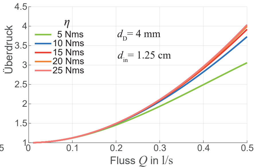
Druck als Funktion Durchfluss Q und Reibungszahl \eta
