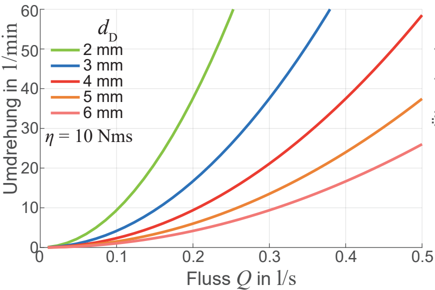
Rotation als Funktion Durchfluss Q und Düsendurchmesser d_D
