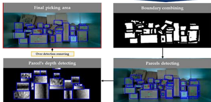
<비전 시스템 전체 플로우 차트>
