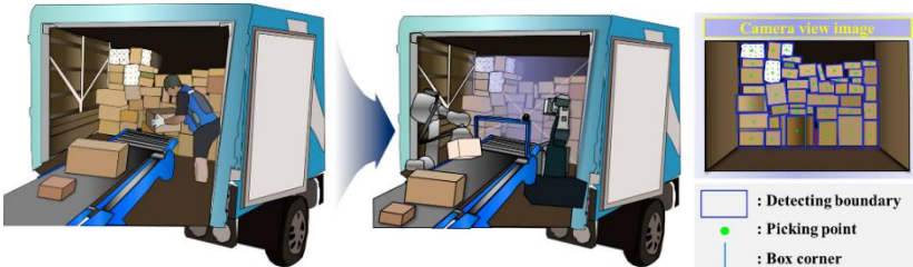
<비전 인식을 통한 자동화 낱소포 하차 시스템>
