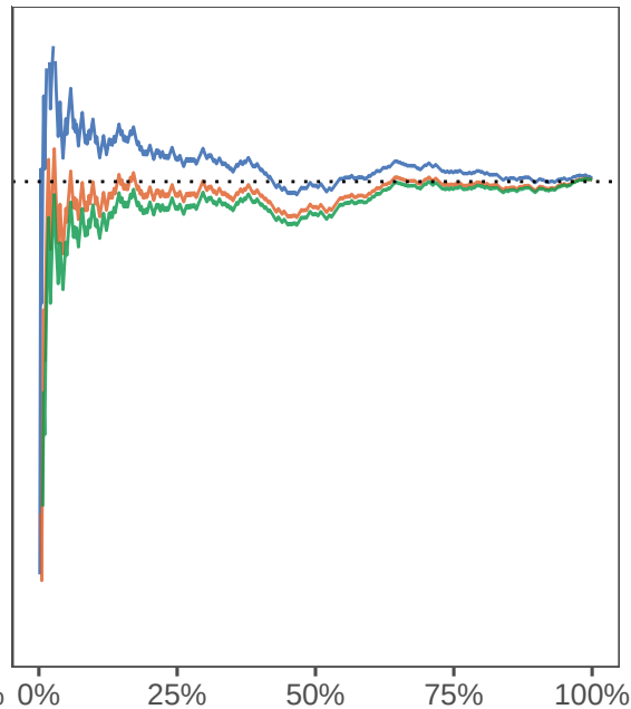
lasso
