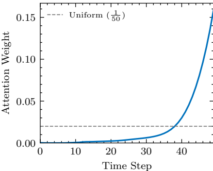
Simple Attention
