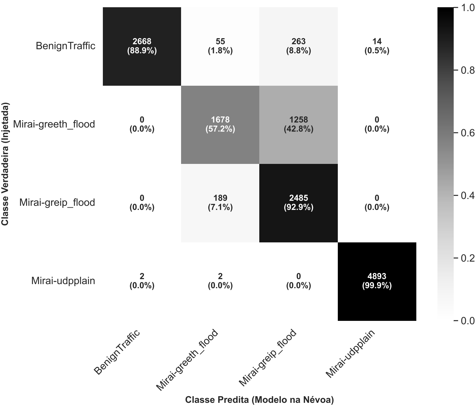
Matriz de Confusão: Classificação Operacional no Testbed 5G
