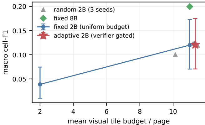
OmniDocBench (n=90)
