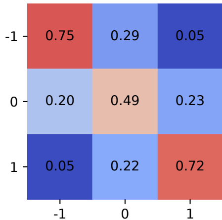
Oligo_NN; n = 2305
