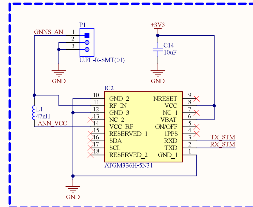
GNSS Module
