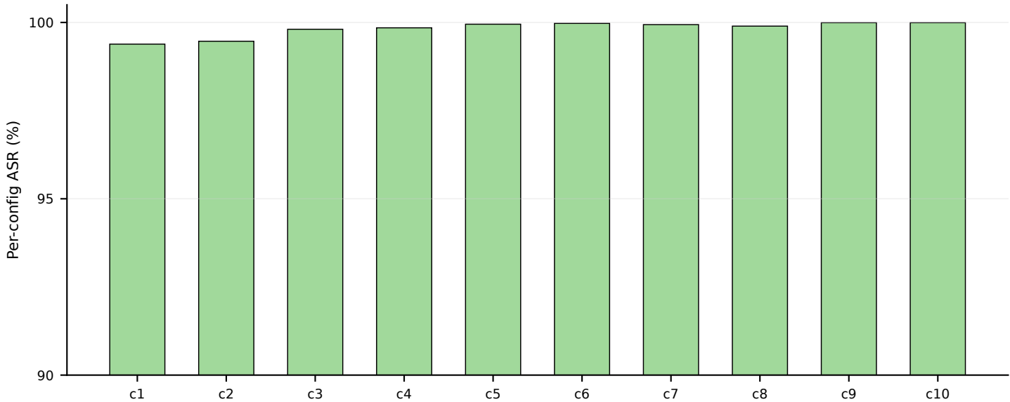
cifar10 / vgg11
