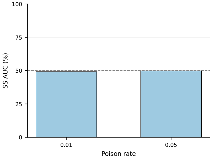
SS AUC
