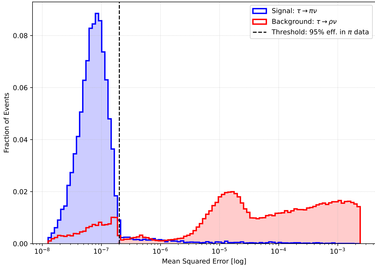
Autoencoder: Anomaly Scores (MSE)
