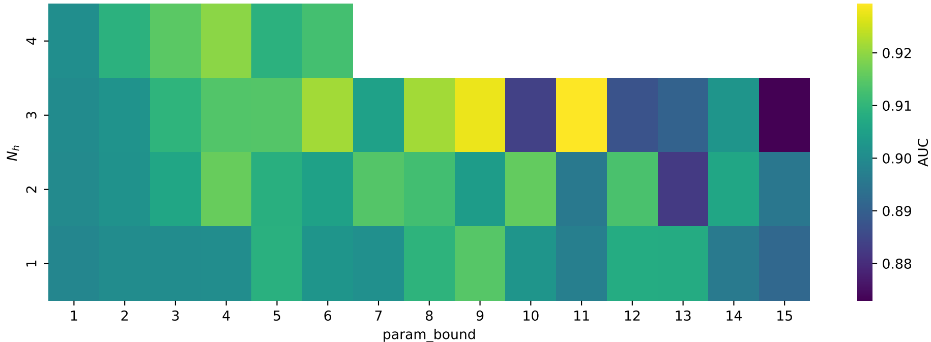
RTBM: Mean AUC - 5 runs , 250 maxiter
