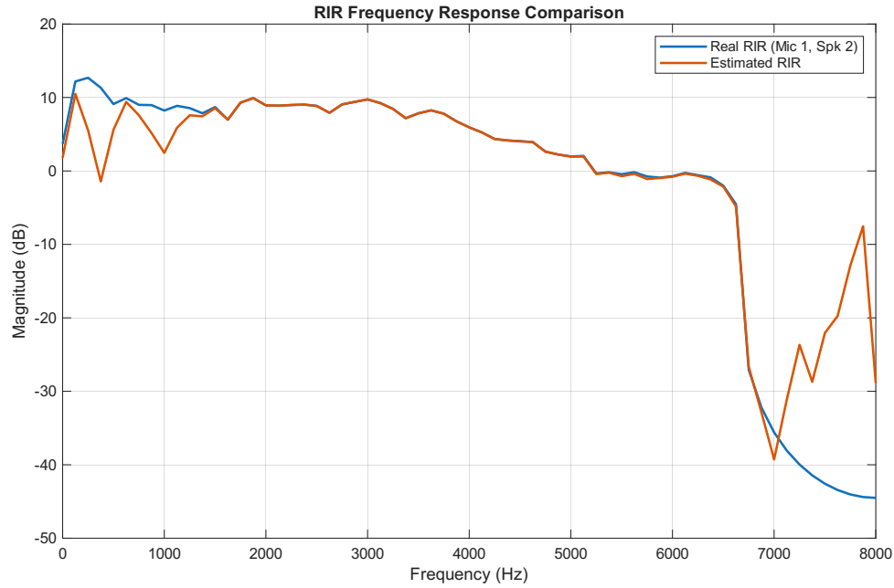
Figura 8: Modulo della trasformata della RIR reale (blu) e stimata (arancio) con ingresso mono replicato sui canali.
