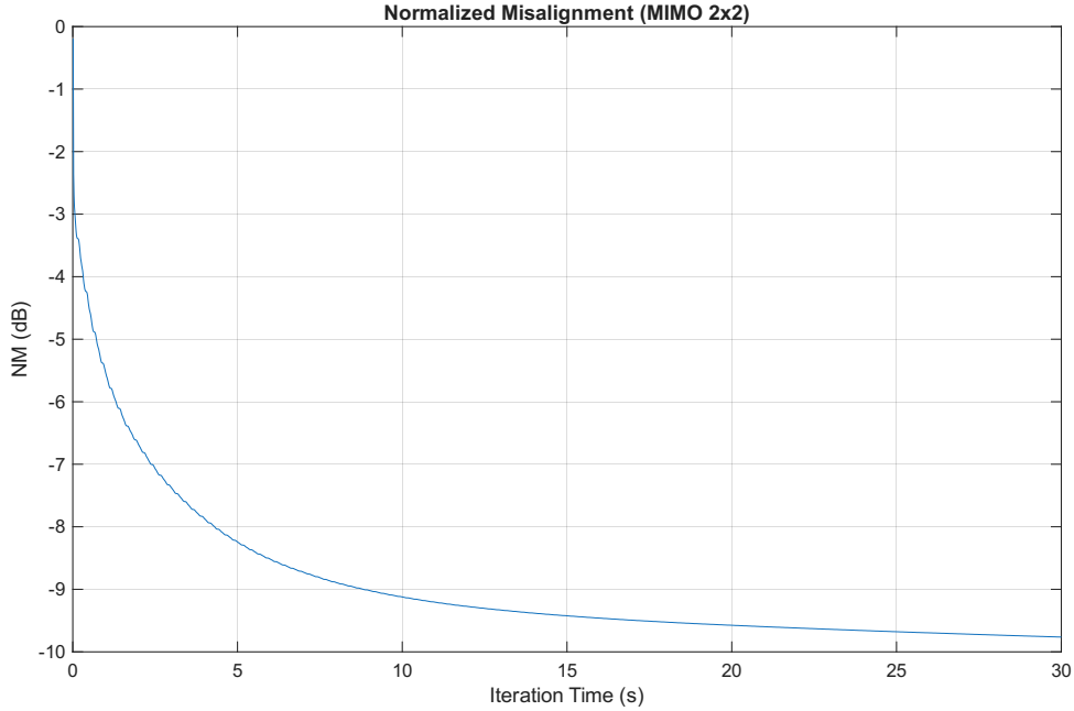
Figura 6: NM nel caso MIMO con canali correlati e decorrelazione tramite modulazione di fase. Frequenza di campionamento f_s = 16 kHz.
