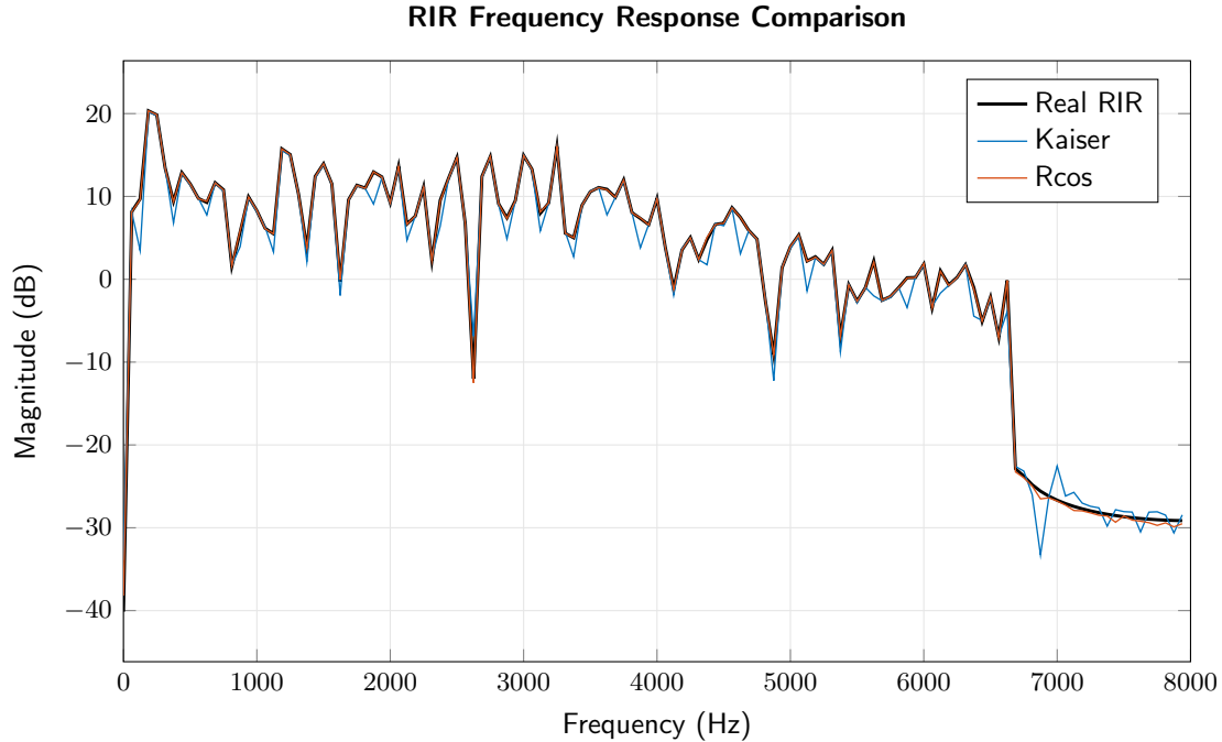
Figura 4: Confronto nel dominio della frequenza tra la RIR reale e le RIR stimate con i due prototipi.
