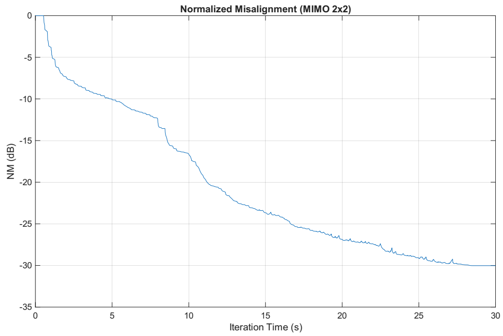
Figura 9: NM nel caso MIMO con ingresso stereo diversificato sui canali.
