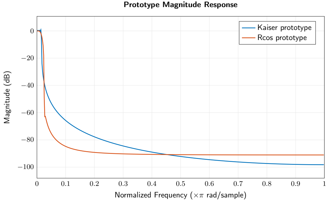
Figura 1: Risposta in frequenza (modulo) dei due prototipi a confronto, entrambi di lunghezza 1025 campioni.
