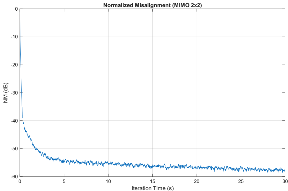
Figura 5: NM nel caso MIMO con ingressi scorrelati (caso ideale). Frequenza di campionamento f_s = 16 kHz.
