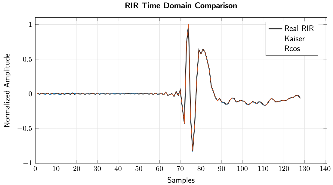
Figura 3: Confronto nel dominio del tempo tra la RIR reale e le RIR stimate con i due prototipi.
