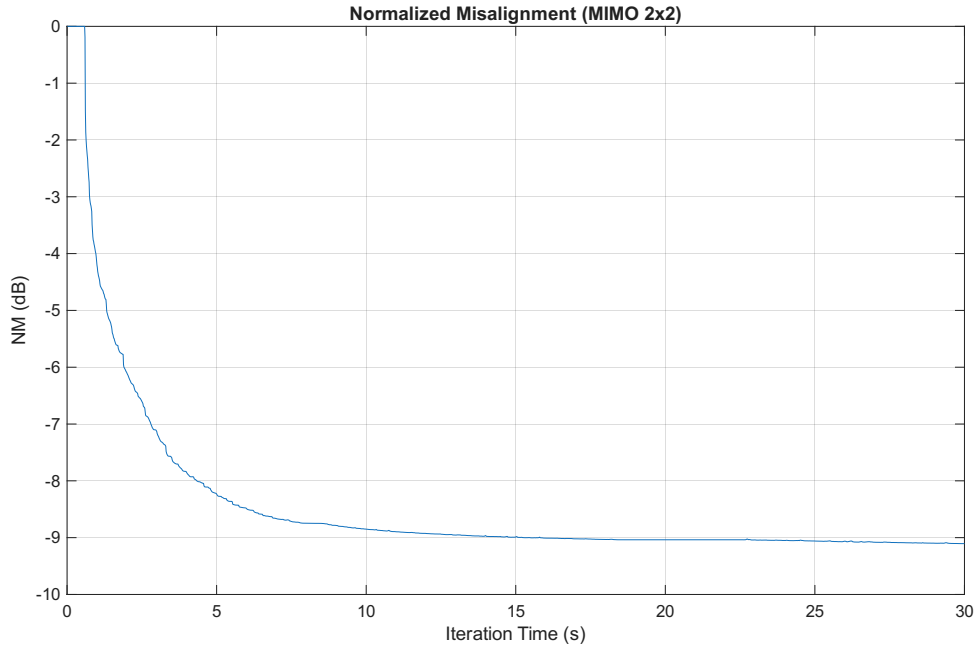
Figura 7: NM nel caso MIMO con ingresso mono replicato sui canali.
