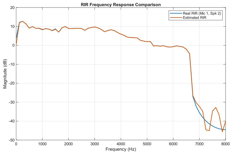
Figura 10: Modulo della trasformata della RIR reale (blu) e stimata (arancio) con ingresso stereo diversificato sui canali.
