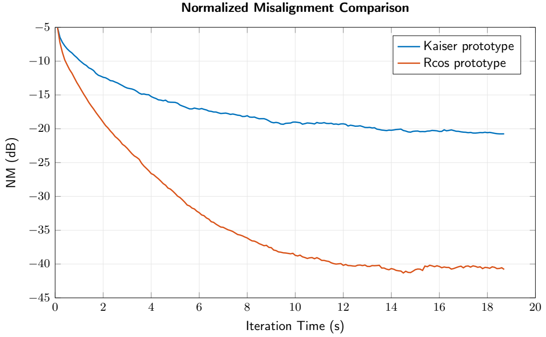
Figura 2: Confronto del normalized misalignment tra i due prototipi, a parità di lunghezza (1025 campioni).
