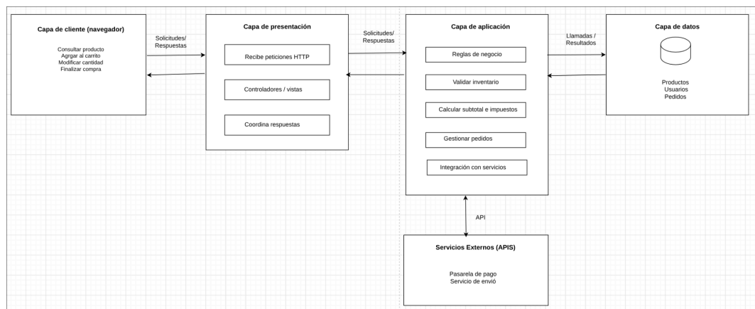
Figura 5: Diagrama del caso de estudio
