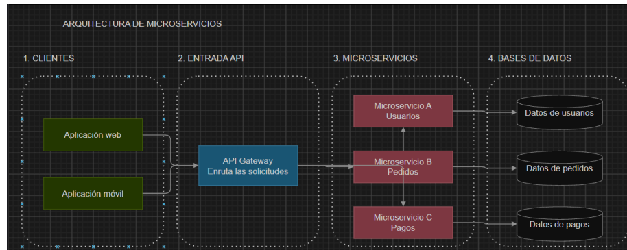
Figura 4: Diagrama de la arquitectura Microservicios
