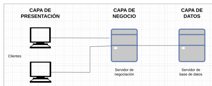
Figura 3: Diagrama de la arquitectura Multicapa
