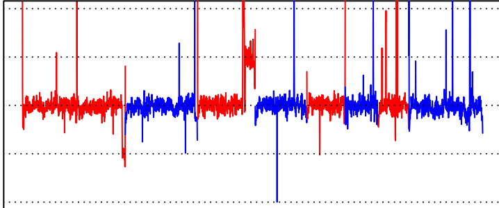
SRR21359696
