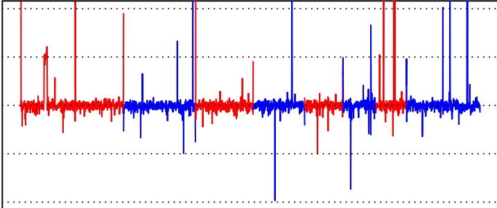
SRR9073716
