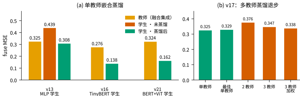
图 3: (a) 单教师嵌合蒸馏: 蒸馏后的学生在每种设置下都超过其多底座教师。(b) 多教师蒸馏在所有配置下退步 (v17)。越低越好。
