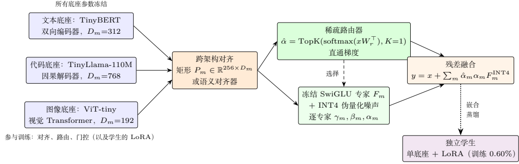
图 1: 异构微观融合与嵌合蒸馏。三个架构与隐藏宽度各异的冻结预训练底座被原生编码, 对齐进共享的 256 维空间, 稀疏路由 ( K=1 ) 到携带 INT4 伪量化噪声的冻结 SwiGLU 专家。嵌合蒸馏随后把集成坍塌为一个独立的单底座学生。
