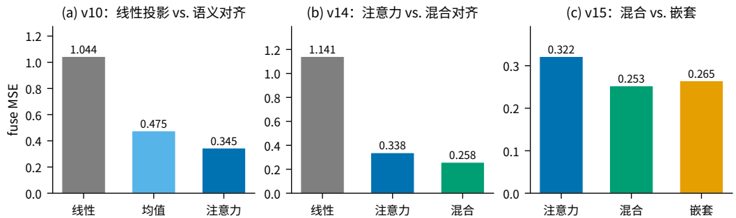
图 2: 对齐器阶梯。(a) 语义对齐优于冻结线性投影, 跨底座注意力优于均值。(b) 混合对齐器优于单概念注意力。(c) 嵌套混合对齐器反而轻微退步: 阶梯在一级跨专家注意力处饱和。越低越好。
