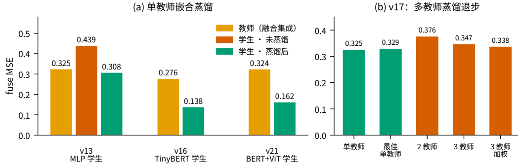
图 6: (a) 单教师嵌合蒸馏: 蒸馏后的学生在每种设置下都超过其多底座教师。(b) 多教师蒸馏在所有配置下退步 (v17)。越低越好。
