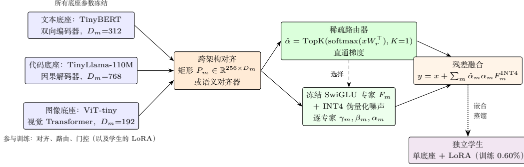
图 2: 异构微观融合与嵌合蒸馏。三个架构与隐藏宽度各异的冻结预训练底座被原生编码, 对齐进共享的 256 维空间, 稀疏路由 ( K=1 ) 到携带 INT4 伪量化噪声的冻结 SwiGLU 专家。嵌合蒸馏随后把集成坍缩为一个独立的单底座学生。
