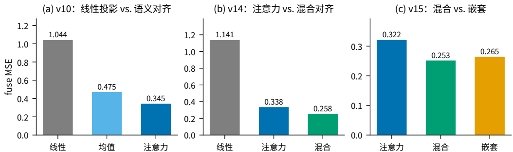
图 5: 对齐器阶梯。(a) 语义对齐优于冻结线性投影, 跨底座注意力优于均值。(b) 混合对齐器优于单概念注意力。(c) 嵌套混合对齐器反而轻微退步: 阶梯在一级跨专家注意力处饱和。越低越好。
