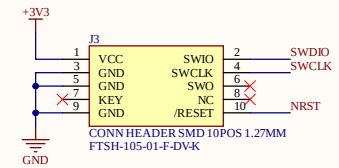
JTAG
