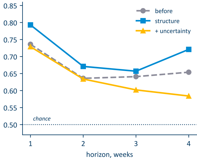
AUC
