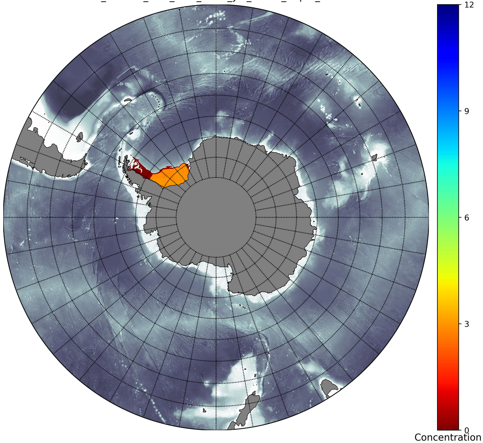
Weddell_TRACER_time_from_58=0_yrs_6mths_Depth_5.8-11.5m
