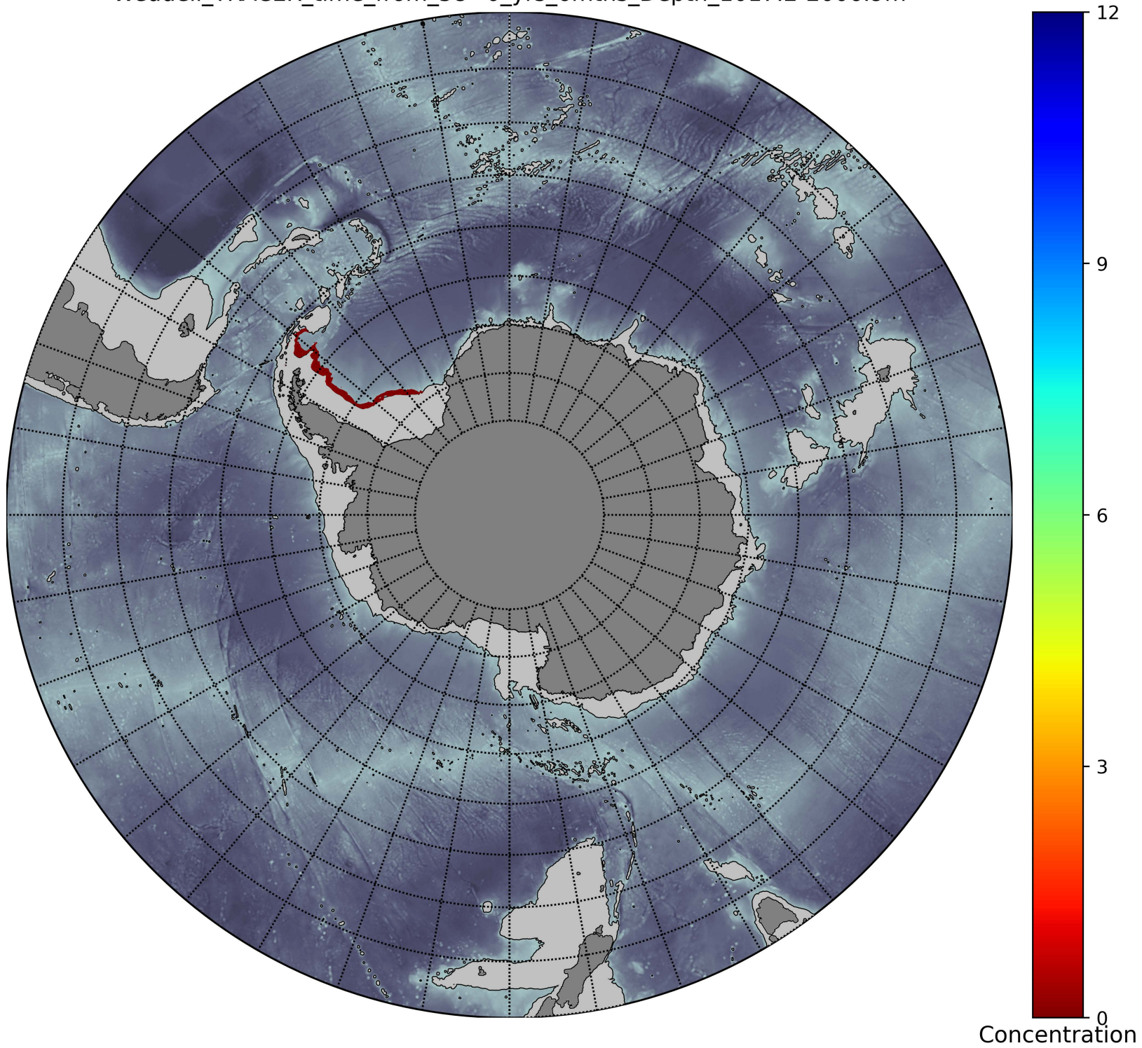
Weddell_TRACER_time_from_58=0_yrs_6mths_Depth_1017.2-2006.9m
