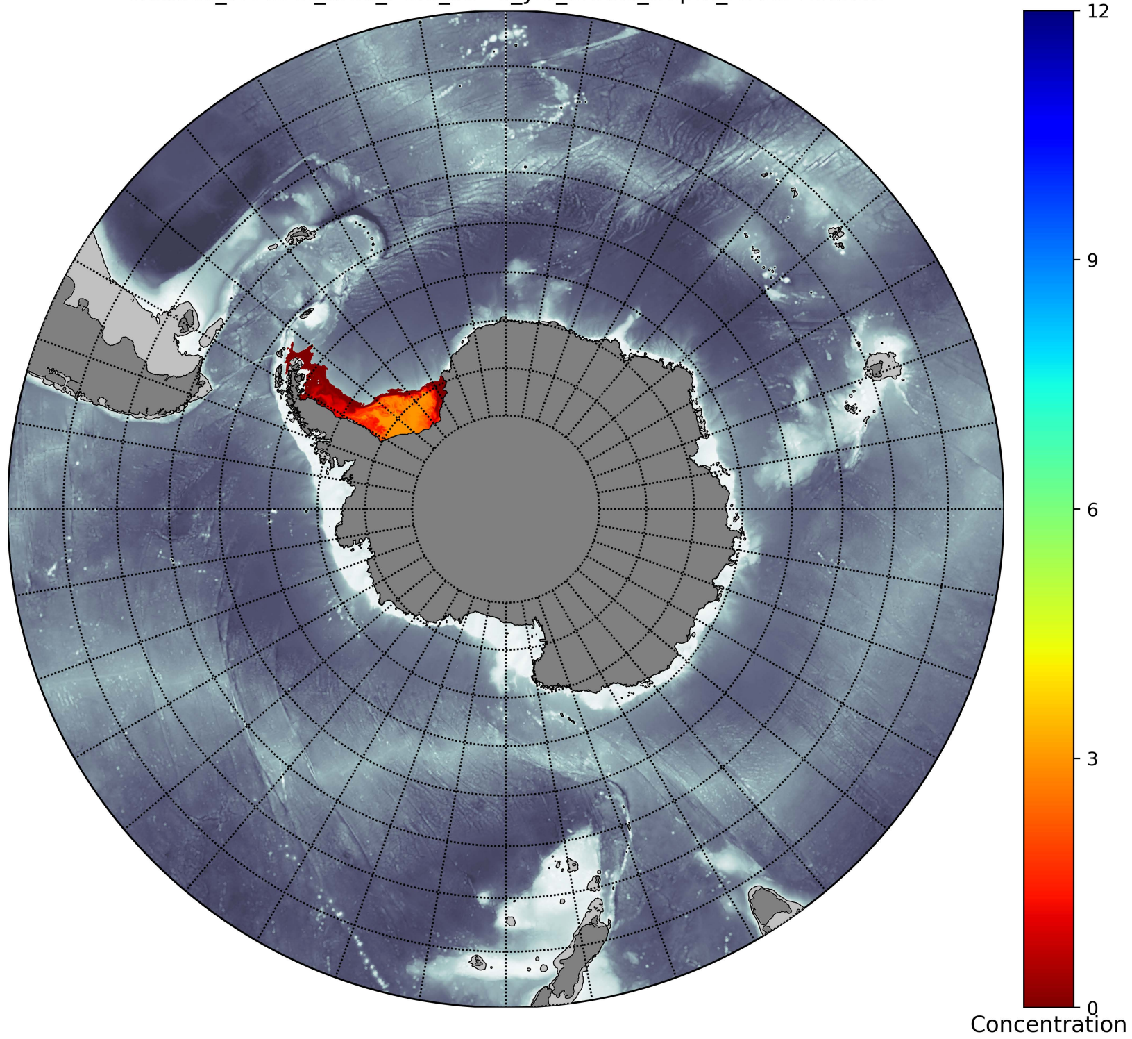
Weddell_TRACER_time_from_58=0_yrs_6mths_Depth_150.5-206.6m
