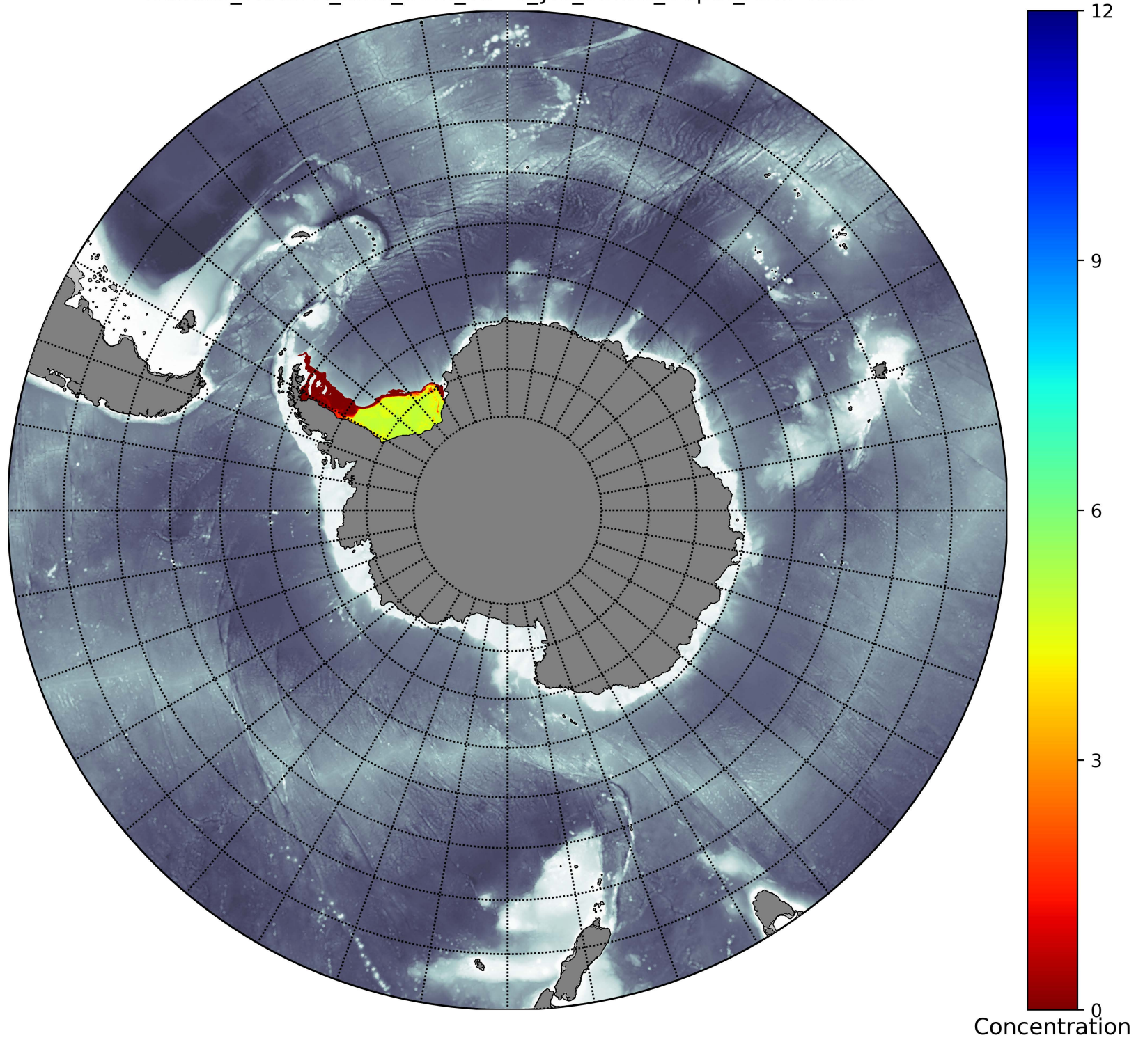
Weddell_TRACER_time_from_58=0_yrs_6mths_Depth_25.6-48.9m
