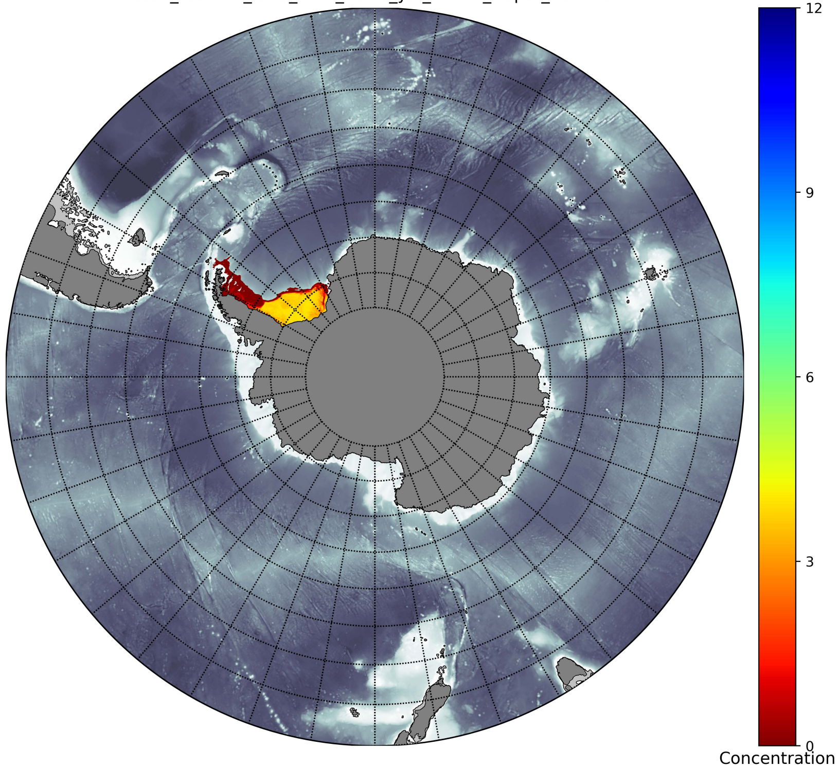
Weddell_TRACER_time_from_58=0_yrs_6mths_Depth_48.9-78.0m
