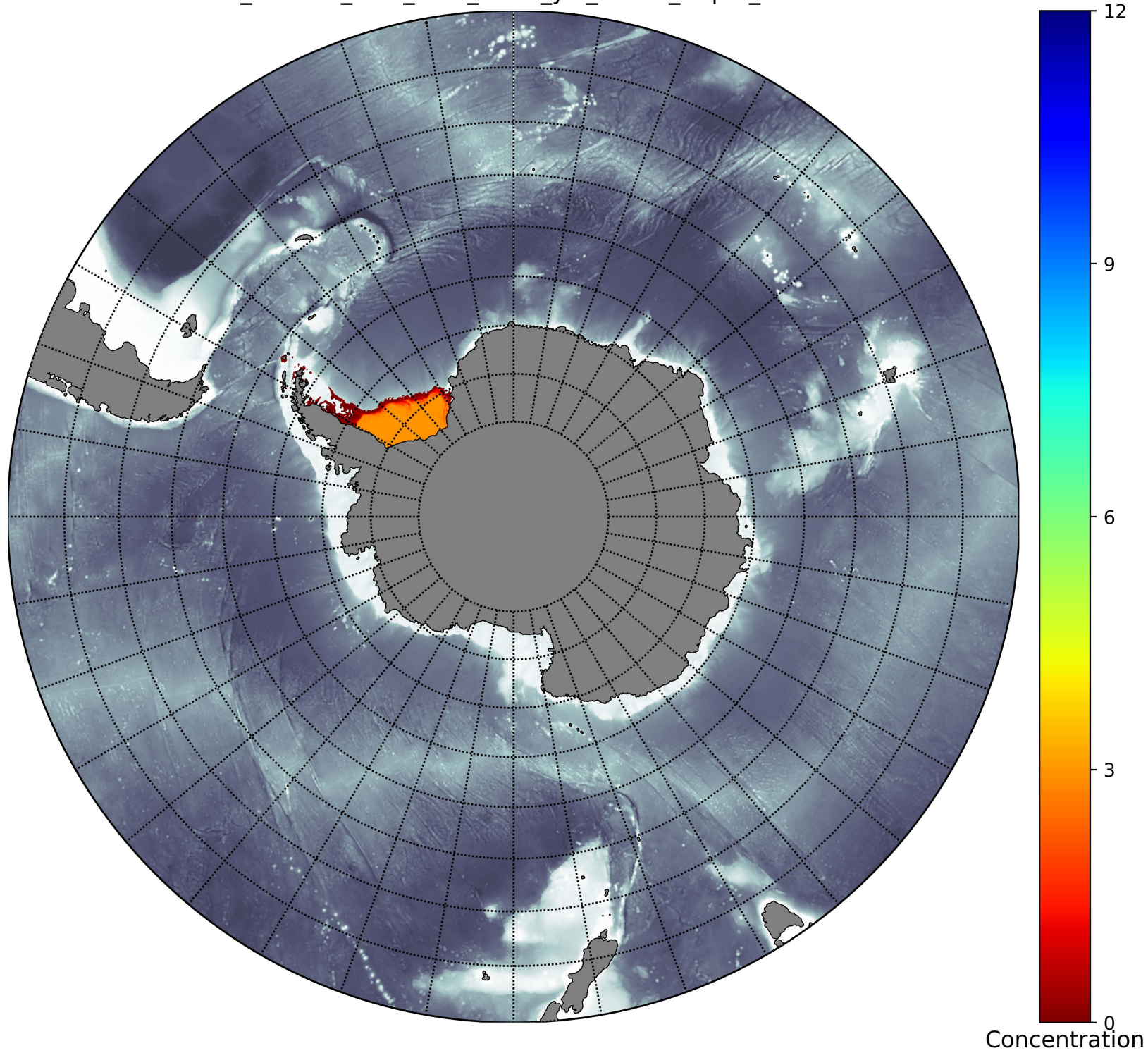
Weddell_TRACER_time_from_58=2_yrs_0mths_Depth_5.8-11.5m
