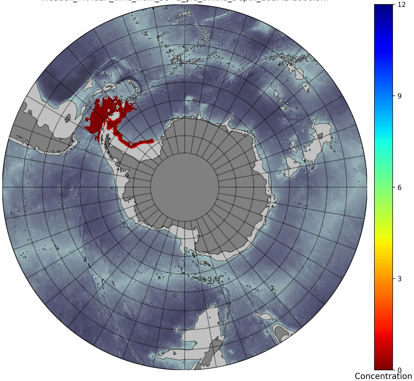
Weddell_TRACER_time_from_58=2_yrs_0mths_Depth_1017.2-2006.9m
