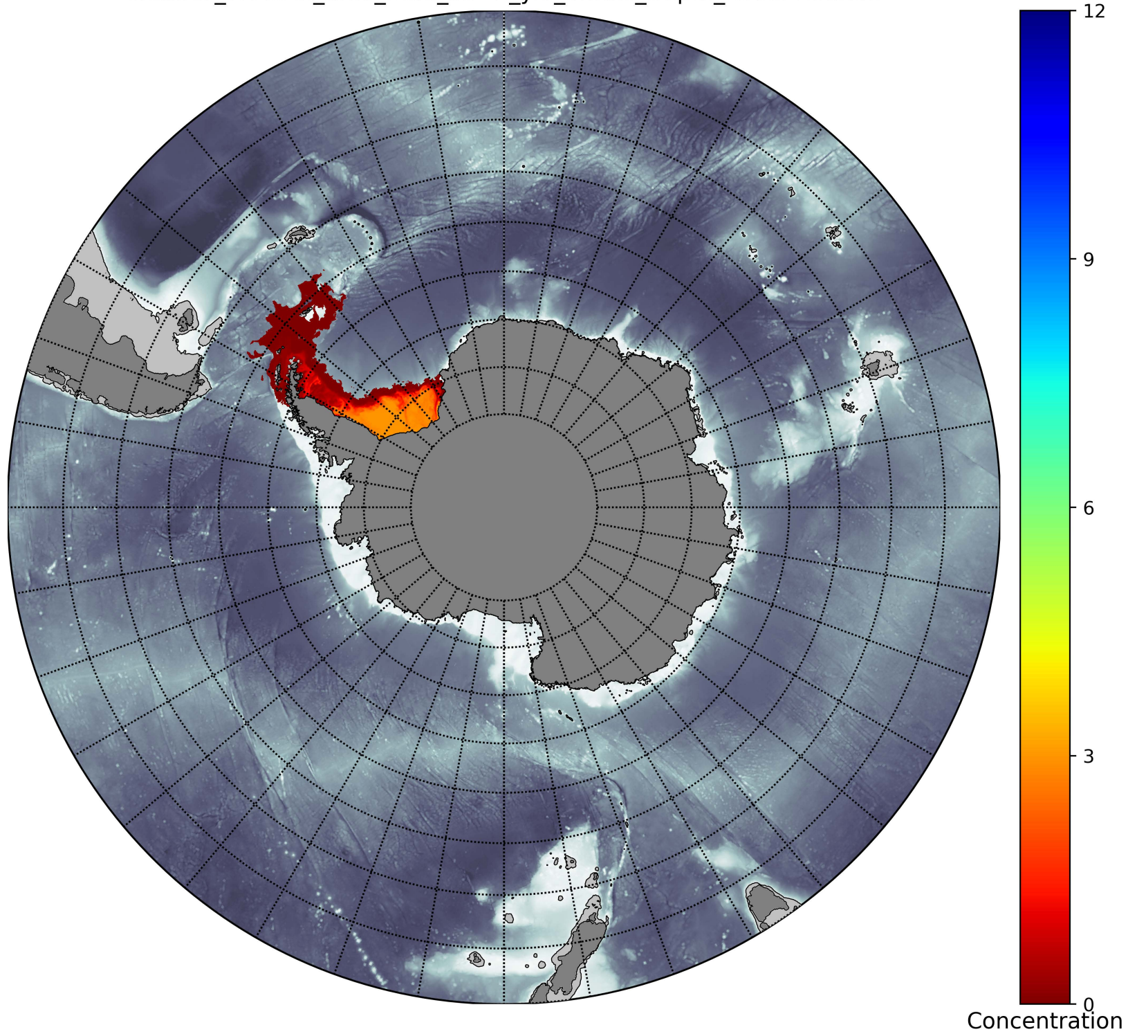
Weddell_TRACER_time_from_58=2_yrs_0mths_Depth_150.5-206.6m
