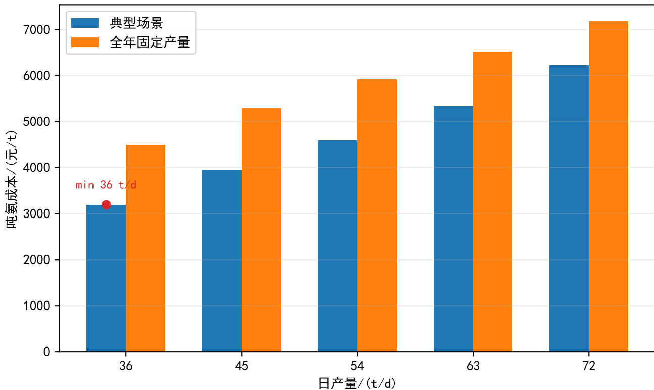
不同日产量吨氨成本比较
