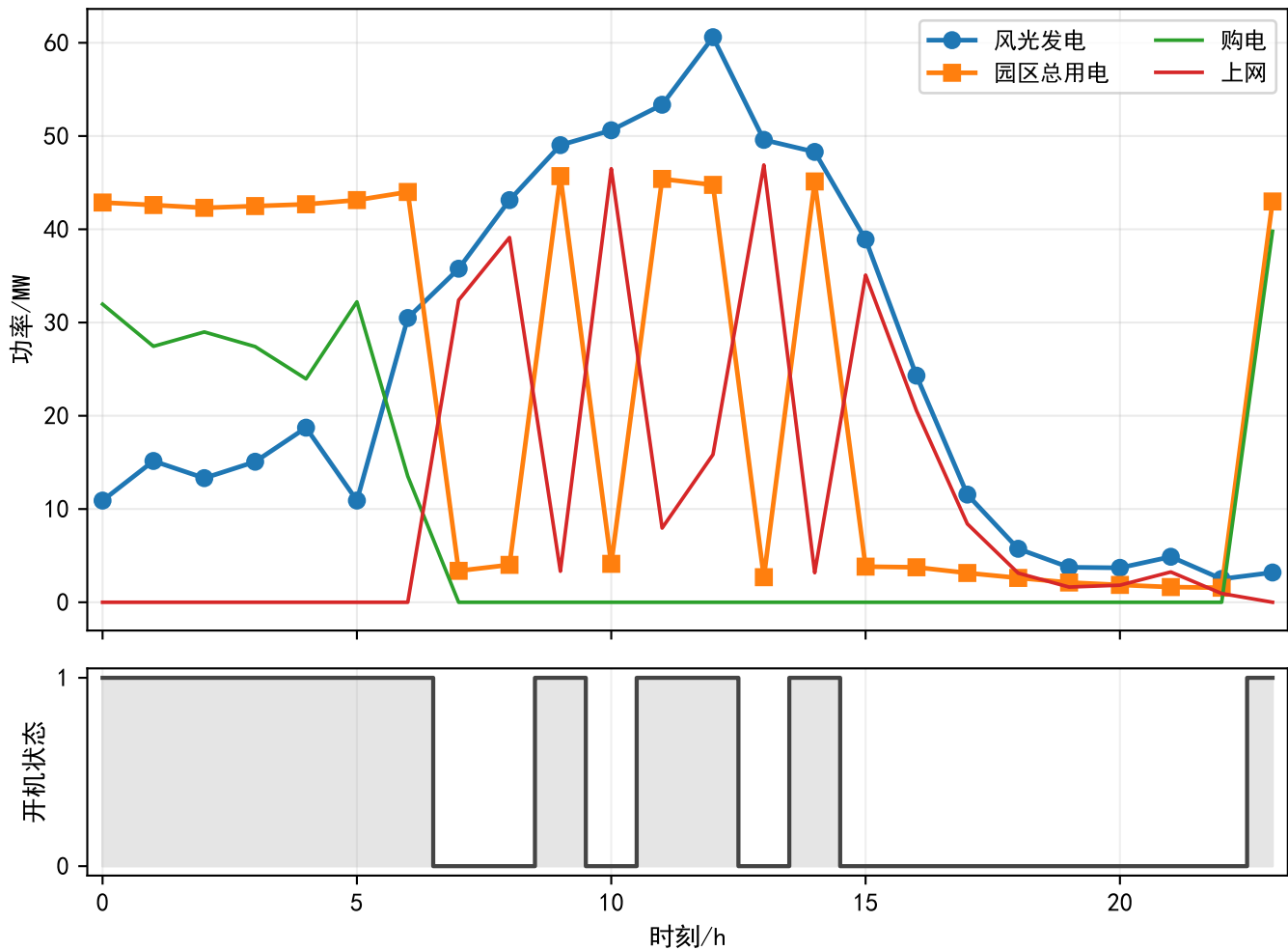
典型场景最低成本方案逐时运行 (36 t/d)
