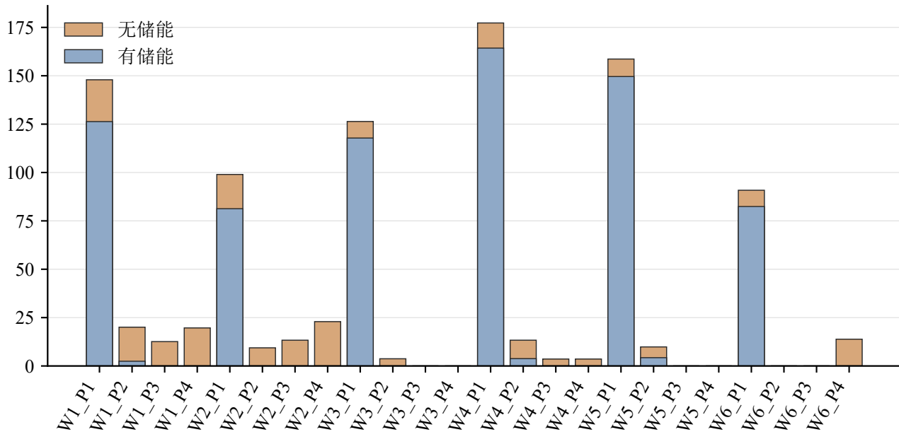
日弃电量 / MWh
