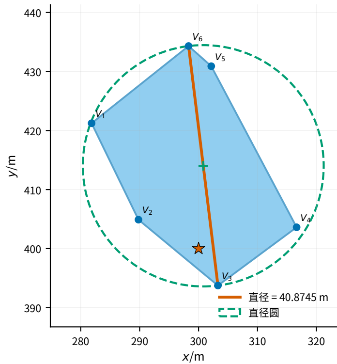
(b) 定位区域、直径端点与直径圆
