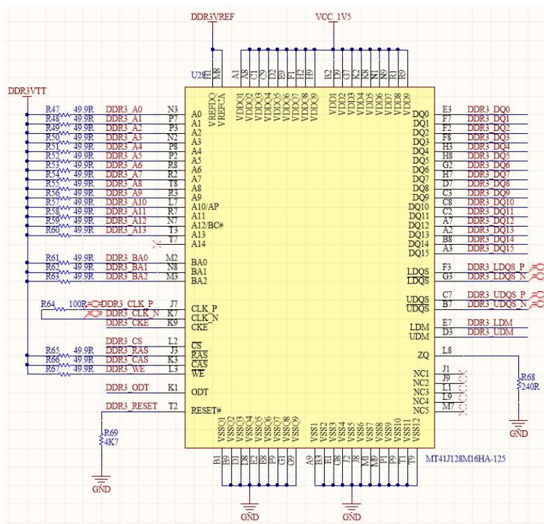
图3-3 DDR3原理图
