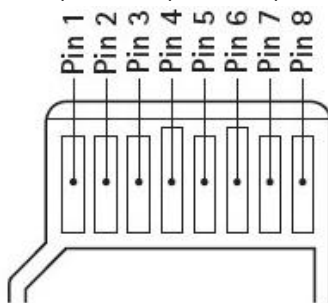
图3-23 SD卡引脚示意图
