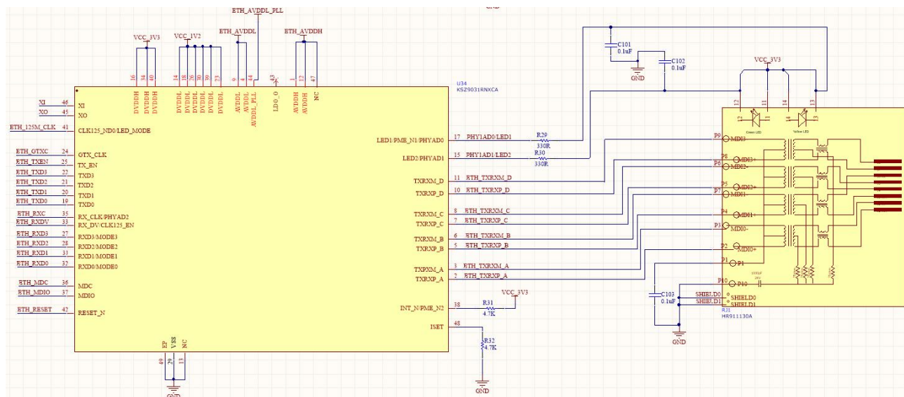
图3-26 以太网接口原理图
