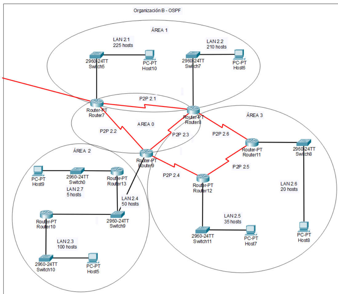
Figura 2. Topología de red de la organización B
