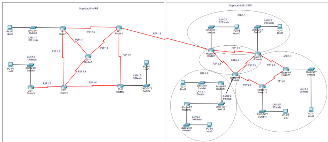
Figura 3. Topología final
