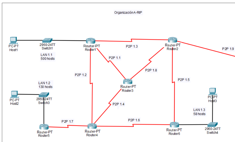
Figura 1. Topología de red de la organización A
