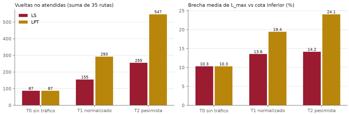
Figura 17: Vueltas no atendidas y brecha media respecto de la cota inferior, por escenario de tráfico.
