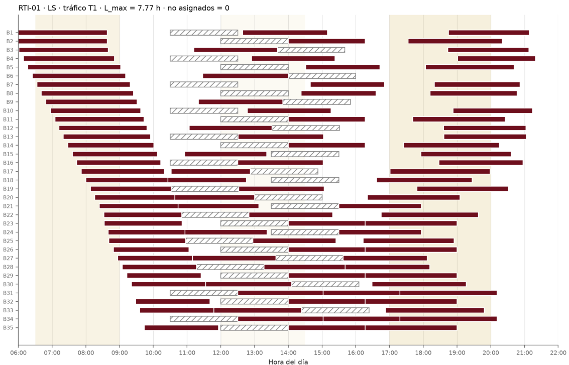
Figura 16: Programa de RTI-01 (35 buses, 103 vueltas) con List Scheduling y tráfico T1.
