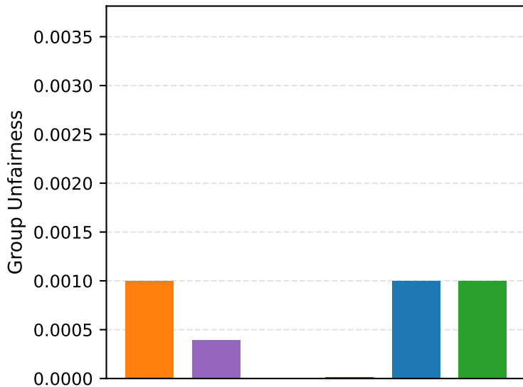
NeuMF
