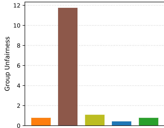
NeuMF
