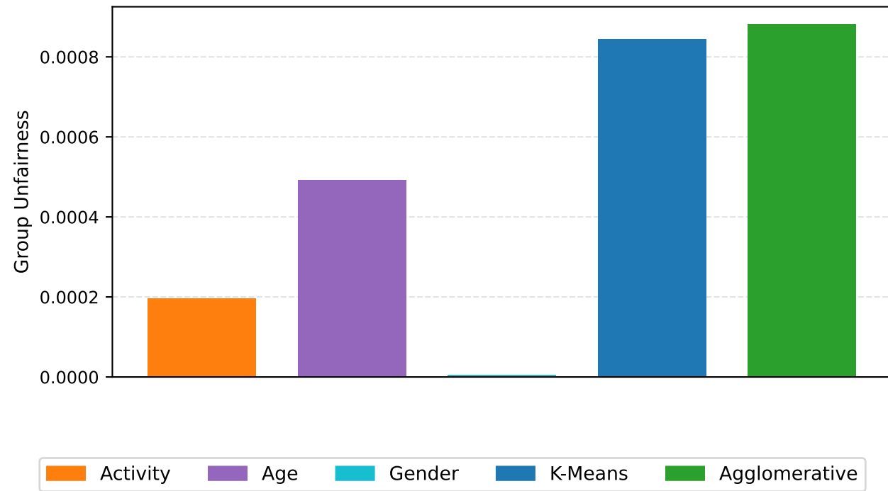
NeuMF
