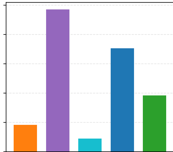
MultiVAE
