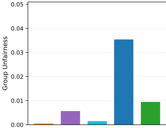
NeuMF
