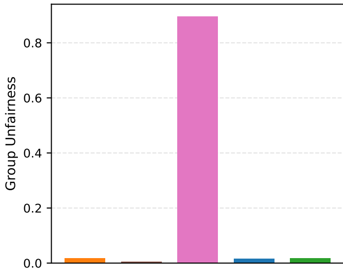
NeuMF
