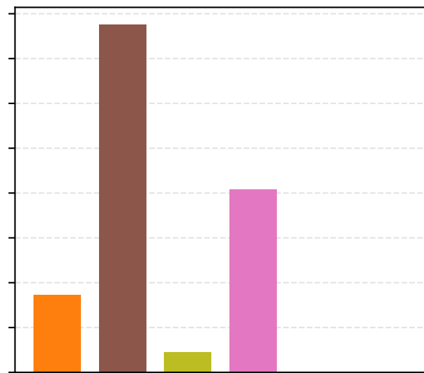
MultiVAE
