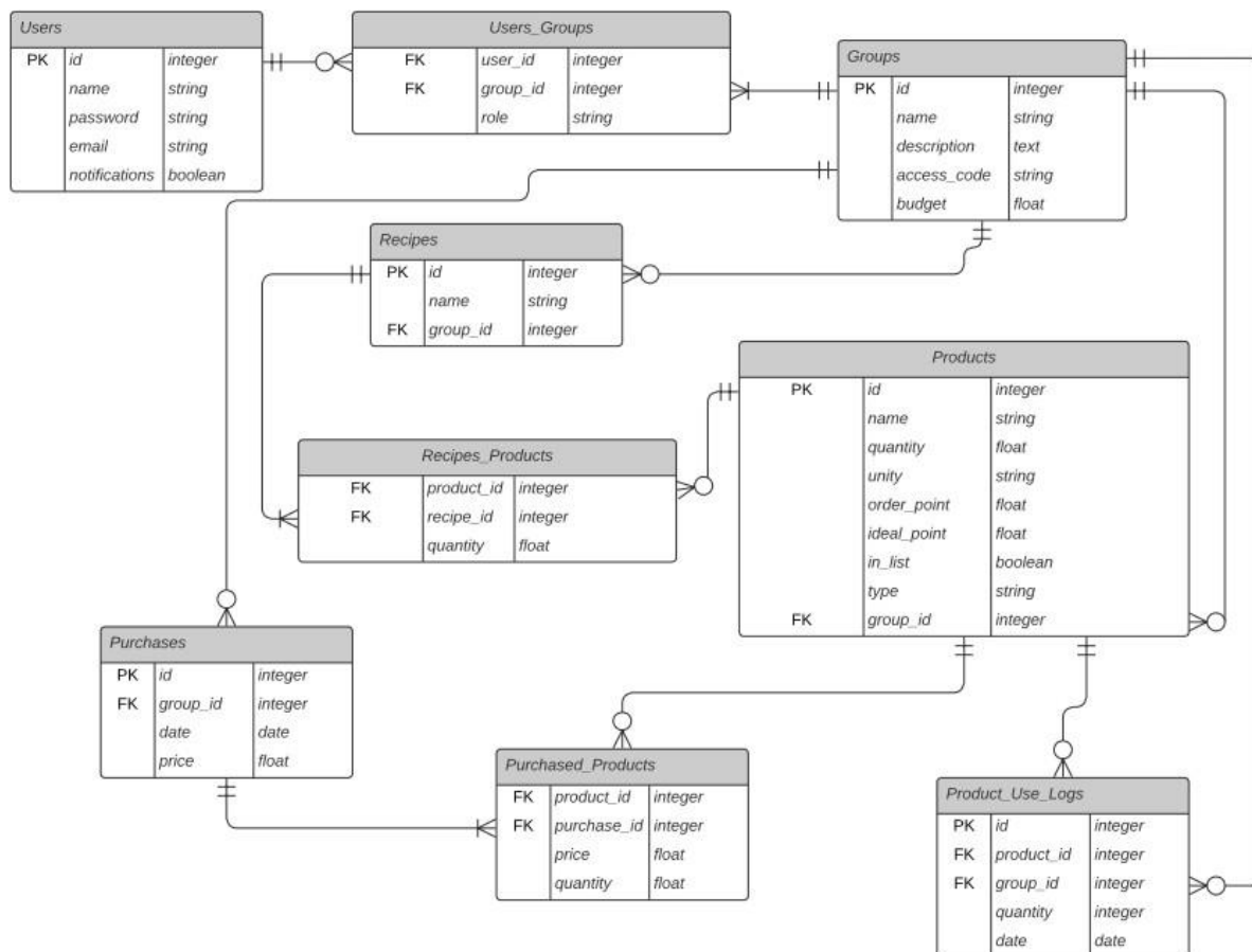
Figura 29 - Diagrama ER
