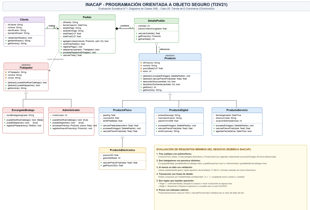
Figura 1: Diagrama de Clases UML - Caso 05: ClickAndGo (archivo editable draw.io disponible en docs/diagrama_clases.drawio).
