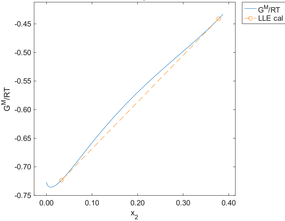
Recta de reparto 4
