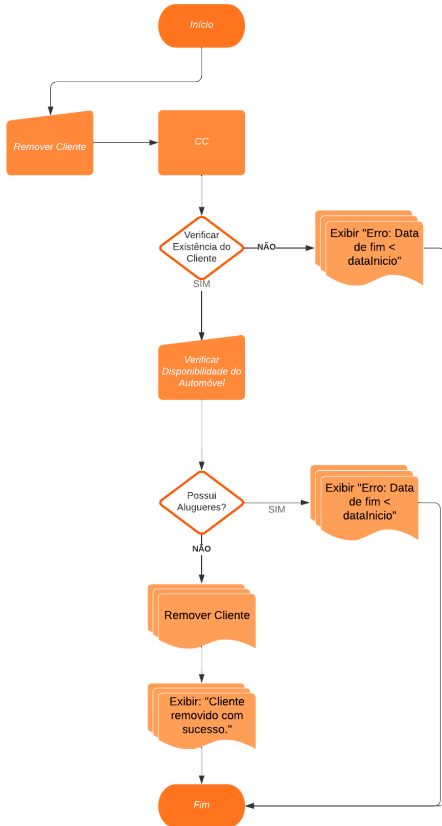
Figura xlvi.: Fluxograma de Remoção de Cliente.
