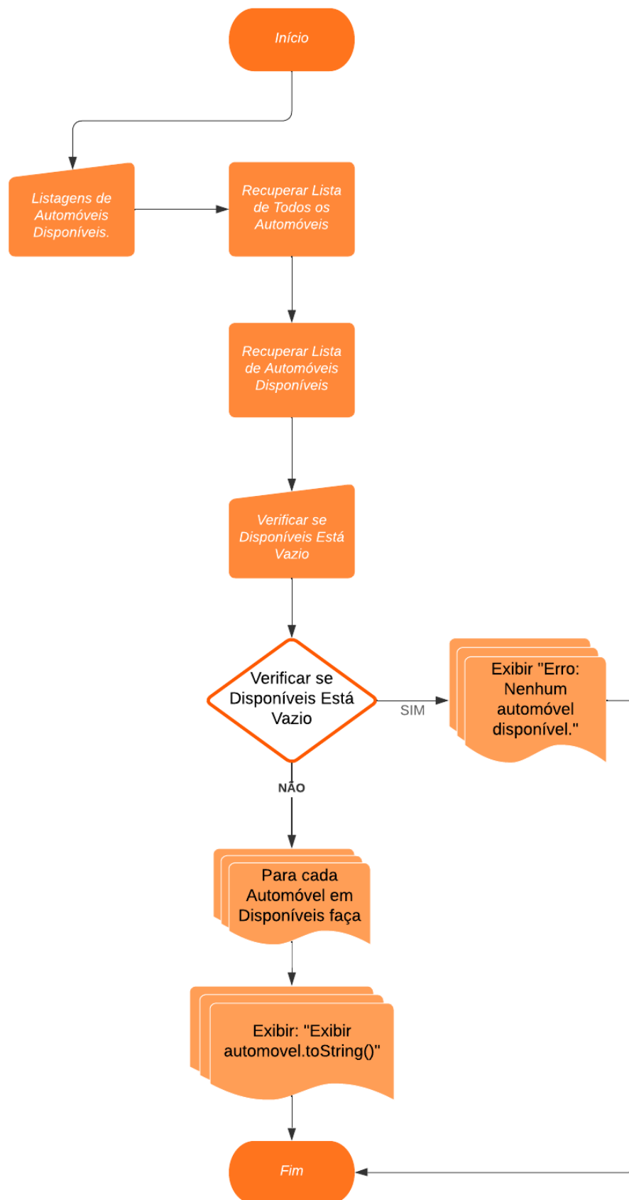
Figura xlix.: Fluxograma de Listagem de Automóveis Disponíveis.
