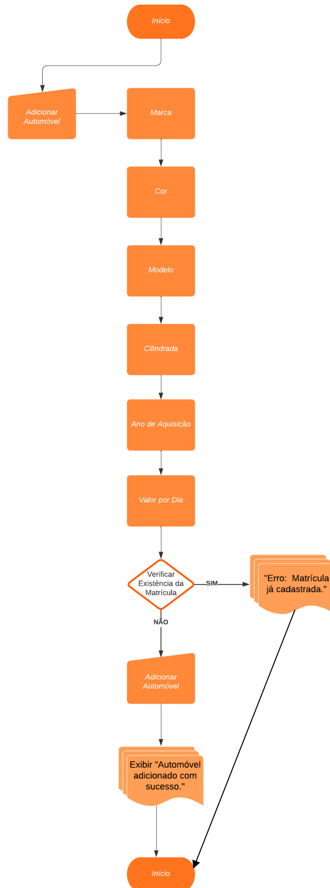
Figura xlv.: Fluxograma de Adição de Automóvel.
