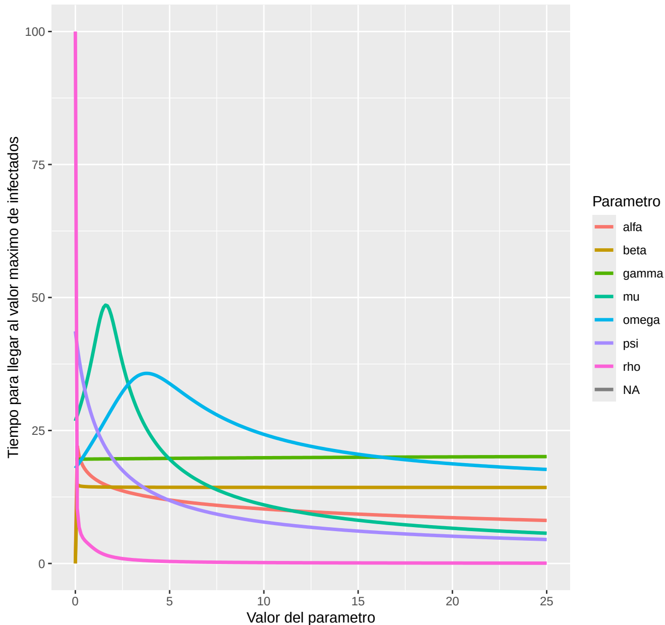
Parametros vs tiempo de valor maximo de infectados
