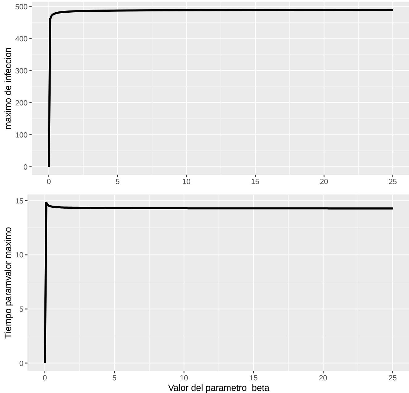
Parametro vs tiempo de valor maximo de infectados para: beta
