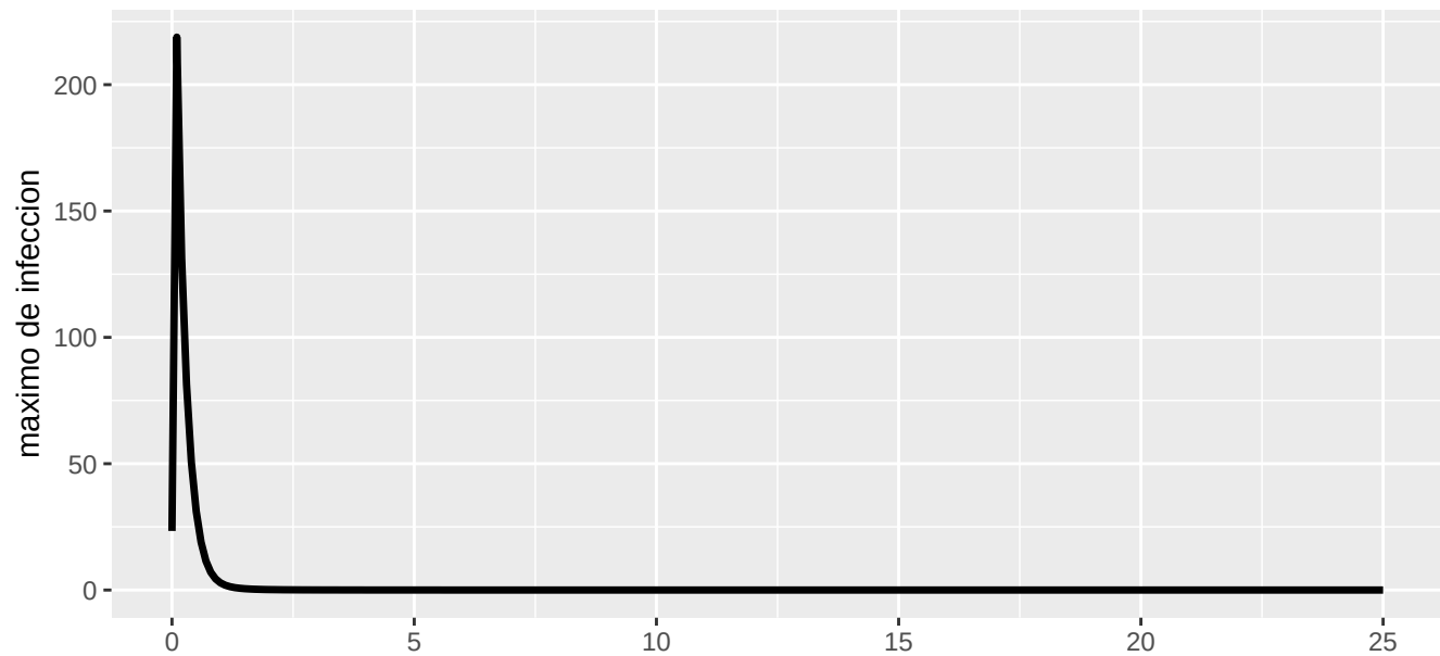
Parametro vs tiempo de valor maximo de infectados para: rho
