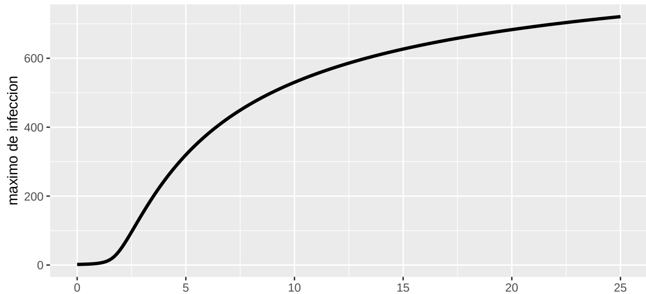
Parametro vs tiempo de valor maximo de infectados para: \mu
