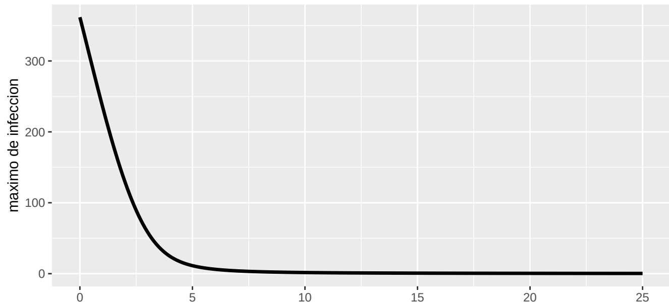
Parametro vs tiempo de valor maximo de infectados para: omega
