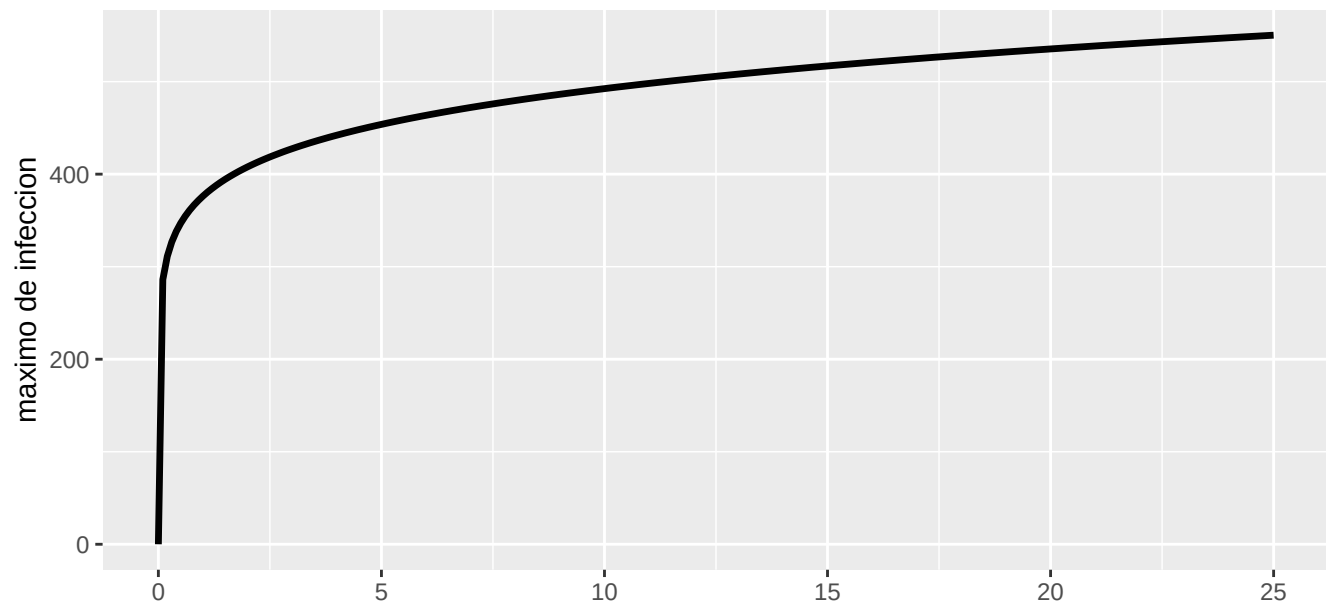
Parametro vs tiempo de valor maximo de infectados para: alfa
