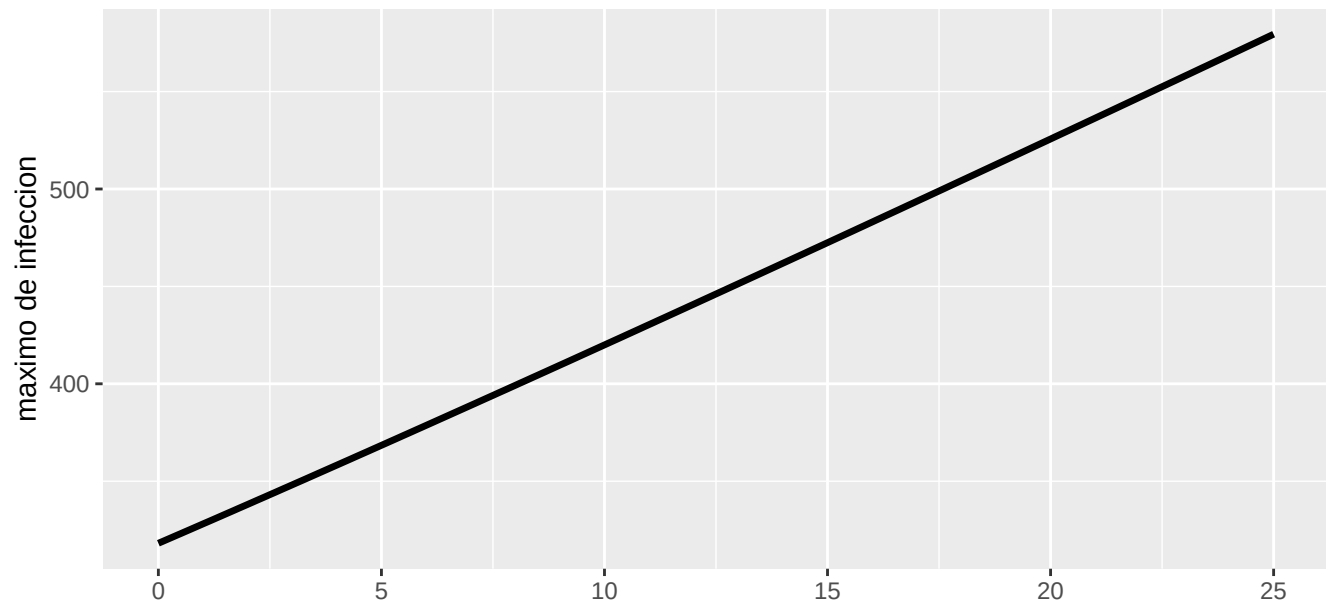
Parametro vs tiempo de valor maximo de infectados para: gamma
