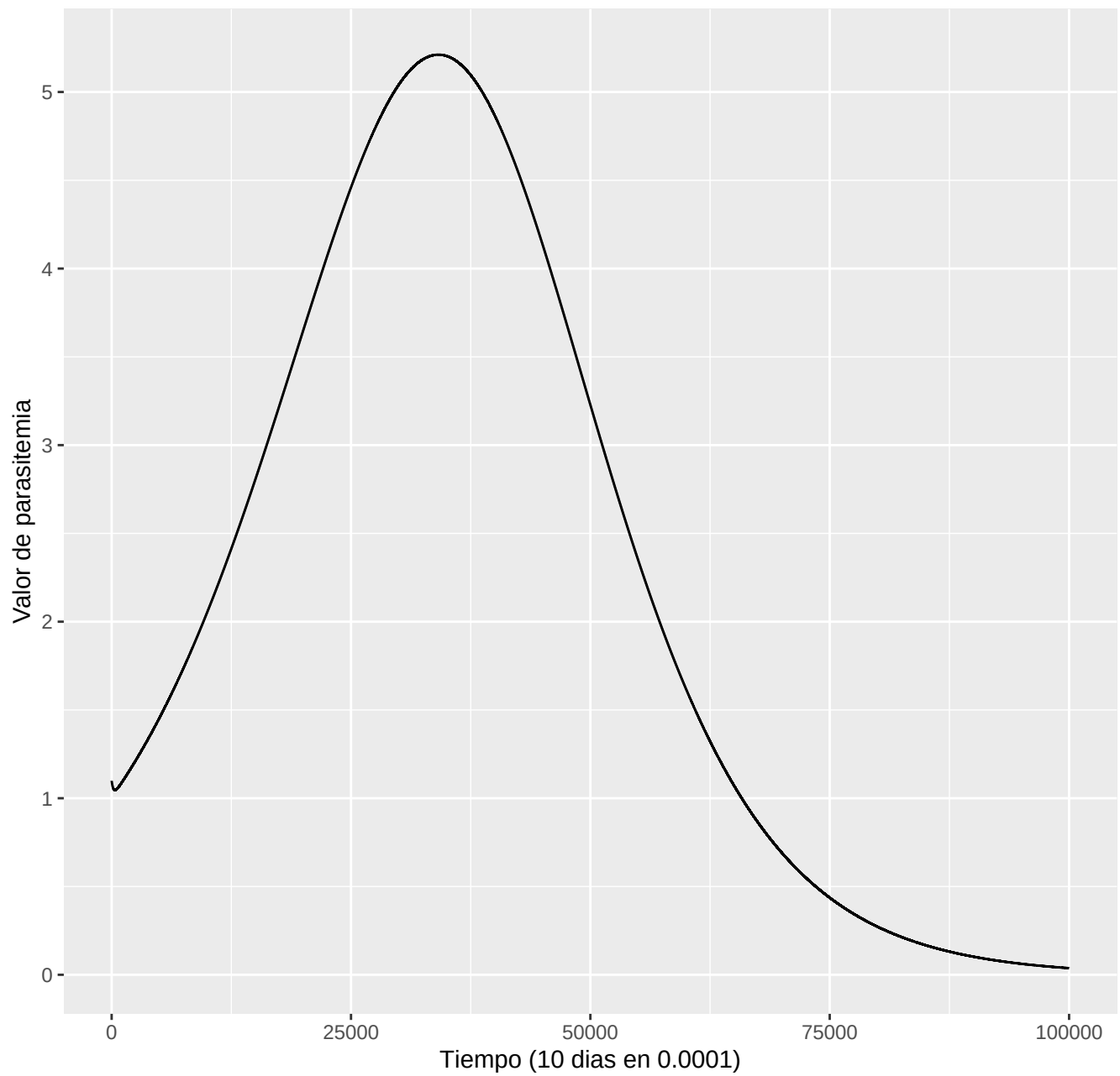
Parasitemia en simulacion
