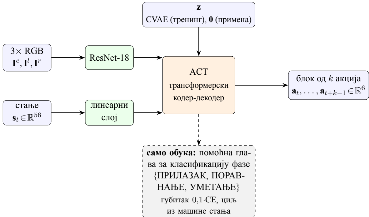
Слика 4: Улазно-излазна шема АСТ политике примењене у овом раду: слике три камере (ResNet-18) и проприоцептивни вектор s_t (линеарни слој), уз латентну променљиву z , улазе у трансформерски кодер-декодер који предвиђа блок од k акција. Испрекидано је приказана помоћна глава за класификацију фазе, активна само у обуци (губитак 0,1-СЕ), чији циљеви (ПРИЛАЗАК/ПОРАВНАЊЕ/УМЕТАЊЕ) потичу из машине стања oracle политике. У фази примене z = 0 и примењује се временско усредњавање.
