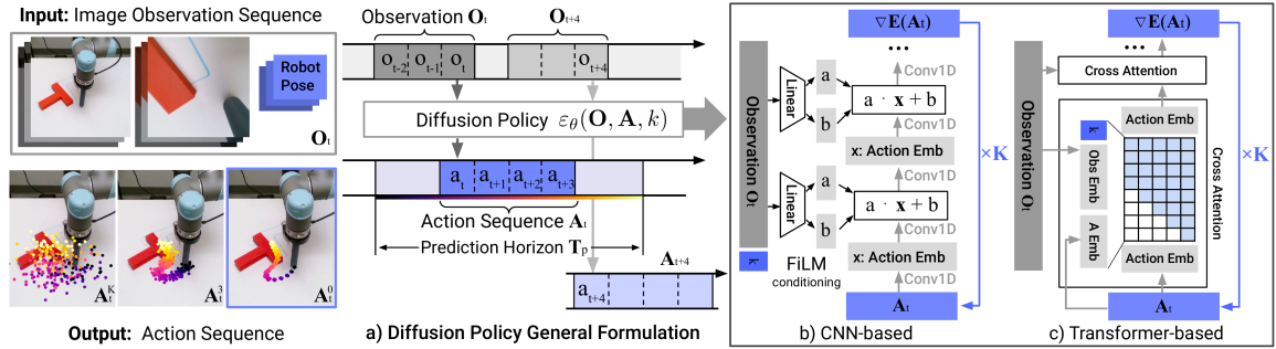
Слика 2: Архитектура Diffusion Policy. Лево је општа формулација: политика \epsilon_\theta(\mathbf{O}, \mathbf{A}, k) узима последњих T_o корака опсервације \mathbf{O}_t и итеративним одшумљавањем зашумљене секвенце ( \mathbf{A}_t^K \rightarrow \mathbf{A}_t^0 , кроз K корака) генерише акције дуж хоризонта предвиђања T_p , од којих се извршава првих T_a . У средини је конволуциона варијанта (Conv-DP): опсервација \mathbf{O}_t FiLM модулацијом ( a\mathbf{x} + b ) условљава Conv1D слојеве мреже за одшумљавање. Десно је трансформерска варијанта (Trans-DP): векторска репрезентација (енгл. embedding ) опсервације улази у унакрсну пажњу сваког декодерског блока уз каузално маскирање пажње. Преузето из [2].
