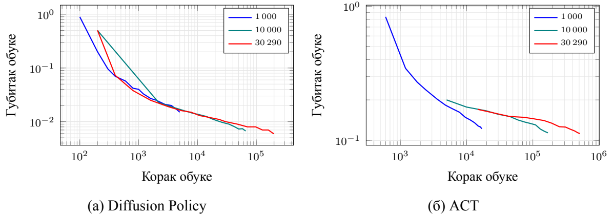
Слика 7: Криве учења (лог–лог скала) за три величине скупа демонстрација. (а) Код Diffusion Policy финални губитак јасно опада са обимом података ( \approx 0,015 \rightarrow 0,007 \rightarrow 0,006 ); ординату чини дифузиони средњеквадратни губитак уз помоћни губитак фазе. (б) Код АСТ-а финални губитак ( L_1 + помоћни губитак фазе) конвергира ка блиском платоу ( \approx 0,122 \rightarrow 0,114 \rightarrow 0,112 ), уз тек благо снижење са обимом података. Апсолутне вредности две ординате нису међусобно упоредиве (различит састав губитка).
