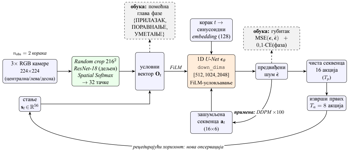
Слика 5: Детаљна архитектура и ток података Diffusion Policy примењене у овом раду. Сlike три камере и проприоцептивно стање (за n_{\text{obs}} = 2 корака) кодирају се дељеним ResNet-18 backbone-ом са просторним softmax-ом (32 тачке) у условни вектор \mathbf{O}_t . Мрежа за одшумљавање ( 1\text{D } U\text{-Net } \epsilon_\theta ) условљена је FiLM модулацијом из \mathbf{O}_t и синусоидном векторском репрезентацијом корака дифузије t , и предвиђа шум \hat{\epsilon} додат на зашумљену акцијску секвенцу \mathbf{a}_t . У обуци се минимизује средња квадратна грешка предвиђеног шума уз помоћни губитак фазе; у примени се поступак понавља 100 пута ( DDPM ) да би се из чистог шума генерисала секвенца од T_p = 16 акција, од којих се извршава првих T_a = 8 (рецидирајући хоризонт).
