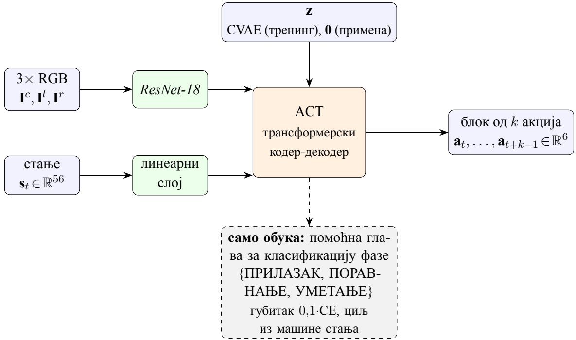
Слика 4: Улазно-излазна шема ACT политике примењене у овом раду: слике три камере ( ResNet-18 ) и проприоцептивни вектор \mathbf{s}_t (линеарни слој), уз латентну променљиву \mathbf{z} , улазе у трансформерски кодер-декодер који предвиђа блок од k акција. Испрекидано је приказана помоћна глава за класификацију фазе, активна само у обуци (губитак 0,1 \cdot \text{CE} ), чији циљеви (ПРИЛАЗАК/ПОРАВНАЊЕ/УМЕТАЊЕ) потичу из машине стања oracle политике. У фази примене \mathbf{z} = \mathbf{0} и примењује се временско усредњавање.
