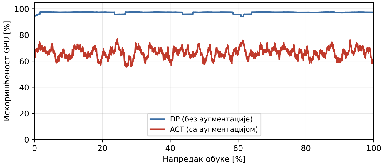
Просечна искоришћеност GPU током обуке на пуном скупу (RTX 5090)
