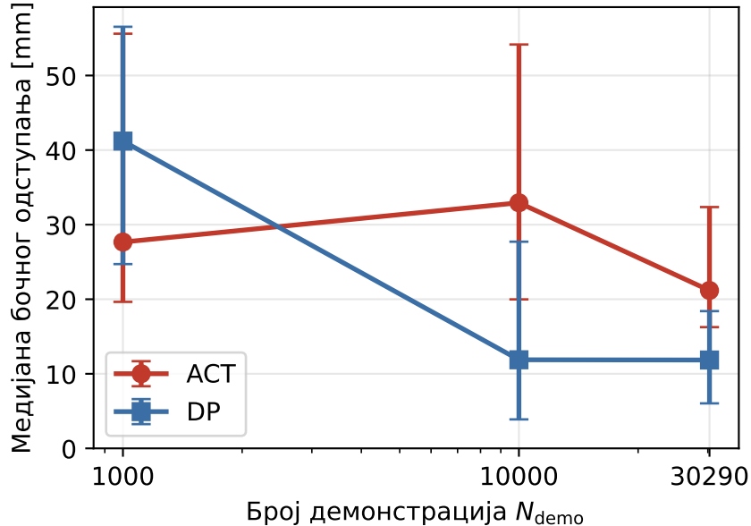
(б) Поравнање са осом
