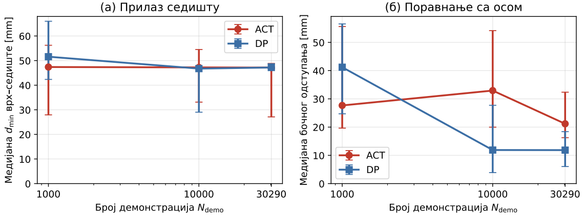
Слика 8: Скалирање прецизности са бројем демонстрација за АСТ и Diffusion Policy ( N = 50 епизода по конфигурацији; тачке су медијане, интервали Q1--Q3). (а) Медијана минималне удаљености d_{\min} врх--седиште остаје на платоу \approx 47 mm, готово независно од обима података и архитектуре. (б) Медијана бочног одступања од осе уметања јасно опада са бројем демонстрација, најизраженије код Diffusion Policy. Стопа успешности је веома ниска у свим тачкама (пилот 0 %, пуне политике реда 1 %), те није приказана.
