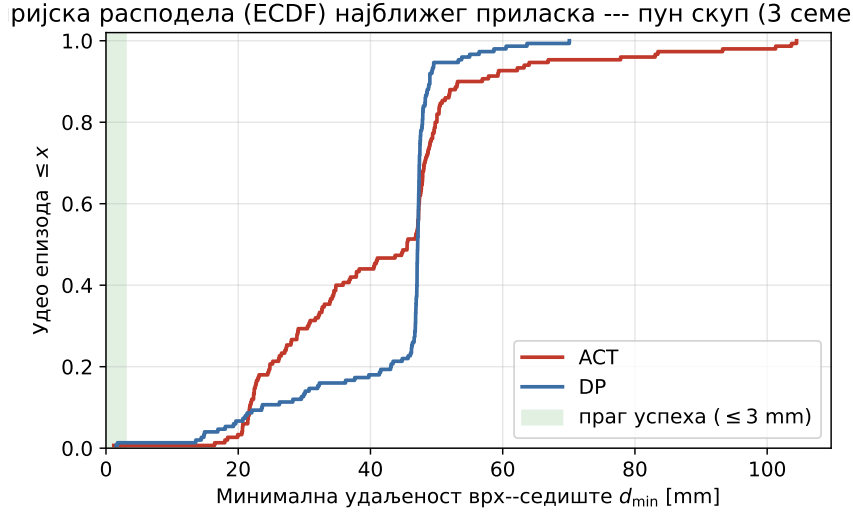
Слика 9: Емпиријска расподела (ECDF) најближег приласка d_{\min} врх--седиште за АСТ и Diffusion Policy обучене на пуном скупу, обједињено преко три семена ( N = 150 епизода по архитектури). Тек мали удео епизода (реда 1 %) досеже праг успешног уметања ( \leq 3 mm, осенчено зелено).
