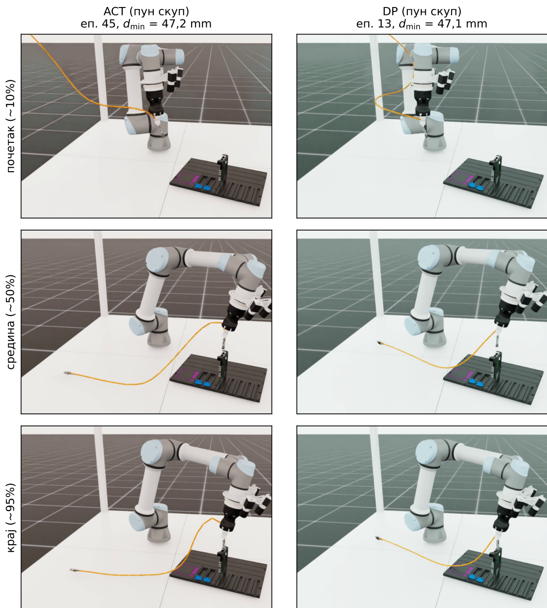
Слика 13: Режим отказа при најбољим конфигурацијама: репрезентативна епизода заустављања за АСТ и Diffusion Policy, три тренутка (~10 %, ~50 %, ~95 % трајања) из погледа трећег лица. Врх конектора долази до близине порта, али уметање се не иницира.
