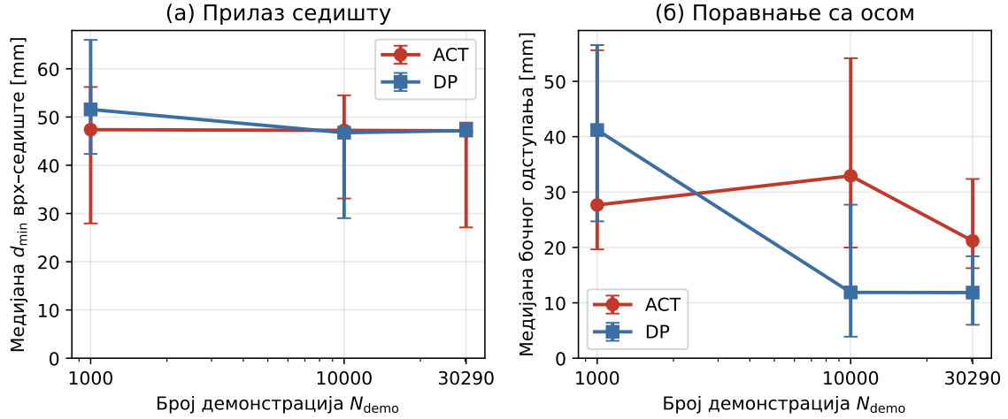
Слика 8: Скалирање прецизности са бројем демонстрација за АСТ и Diffusion Policy ( N = 50 епизода по конфигурацији; тачке су медијане, интервали Q1--Q3). (а) Медијана минималне удаљености d_{\min} врх–лежиште остаје на платоу \approx 47 mm, готово независно од обима података и архитектуре. (б) Медијана бочног одступања од осе уметања јасно опада са бројем демонстрација, најизраженије код Diffusion Policy. Стопа успешности је веома ниска у свим тачкама (пилот 0 %, пуне политике реда 1 %), те није приказана.
