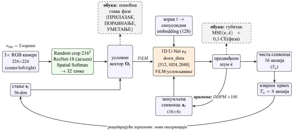
Слика 5: Детаљна архитектура и ток података Diffusion Policy примењене у овом раду. Сlike три камере и проприоцептивно стање (за n_{\text{obs}} = 2 корака) кодирају се дељеном ResNet-18 кичмом са просторним softmax-ом (32 тачке) у условни вектор \mathbf{O}_t . Мрежа за одшумљавање (1D U-Net \epsilon_\theta ) условљена је FiLM модулацијом из \mathbf{O}_t и синусоидним ембедингом корака дифузије t , и предвиђа шум \hat{\epsilon} додат на зашумљену акцијску секвенцу \mathbf{a}_t . У обуци се минимизује средња квадратна грешка предвиђеног шума уз помоћни губитак фазе; у примени се поступак понавља 100 пута (DDPM) да би се из чистог шума генерисала секвенца од T_p = 16 акција, од којих се извршава првих T_a = 8 (рецедирајући хоризонт).
