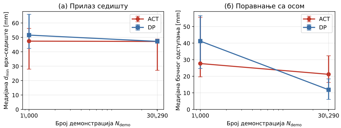
Слика 7: Скалирање прецизности са бројем демонстрација за АСТ и Diffusion Policy ( N = 50 епизода по конфигурацији; тачке су медијане, интервали Q1--Q3). (а) Медијана минималне удаљености d_{\min} врх--седиште остаје на платоу \approx 47 mm, готово независно од обима података и архитектуре. (б) Медијана бочног одступања од осе уметања јасно опада са бројем демонстрација, најизраженије код Diffusion Policy. Стопа успешности је 0 за све конфигурације, те није приказана.
