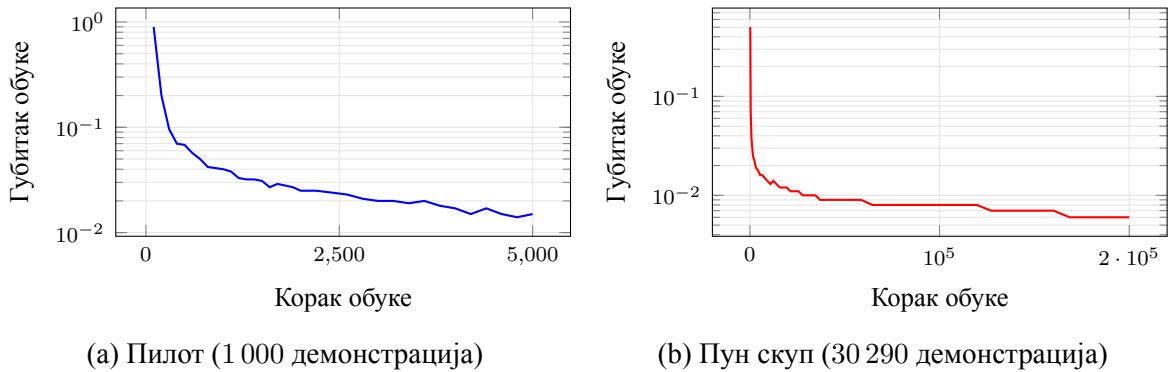
Слика 6: Криве учења Diffusion Policy политике (логаритамска ордината): пилот обука на подскупу и обука на пуном скупу демонстрација.
