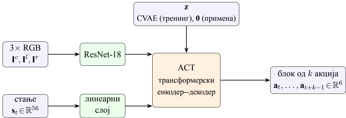
Слика 4: Улазно-излазна шема АСТ политике примењене у овом раду: слике три камере (ResNet-18) и проприоцептивни вектор s_t (линеарни слој), уз латентну променљиву z , улазе у трансформерски енкодер--декодер који предвиђа блок од k акција. У фази примене z = \mathbf{0} и примењује се временско усредњавање.
