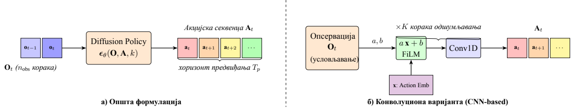
Слика 2: Архитектура Diffusion Policy. (а) Општа формулација: политика \epsilon_\theta(\mathbf{O}, \mathbf{A}, k) условљена опсервацијом \mathbf{O}_t итеративним одшумљавањем генерише акцијску секвенцу \mathbf{A}_t дуж хоризонта предвиђања T_p . (б) Коришћена конволуциона варијанта: опсервација \mathbf{O}_t FiLM модулацијом (a \mathbf{x} + b) условљава Conv1D блокове 1D U-Net-a, кроз K корака одшумљавања.
