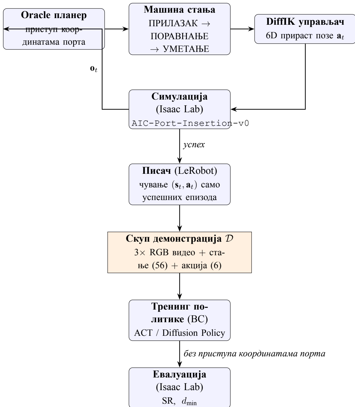
Слика 3: Ток података кроз систем: oracle политика са приступом координатама порта генерише демонстрације преко машине стања и DiffIK управљача, успешне епизоде се чувају у LeRobot скуп демонстрација, на коме се тренирају АСТ и Diffusion Policy политике, а потом евалуирају без привилеговане информације.
