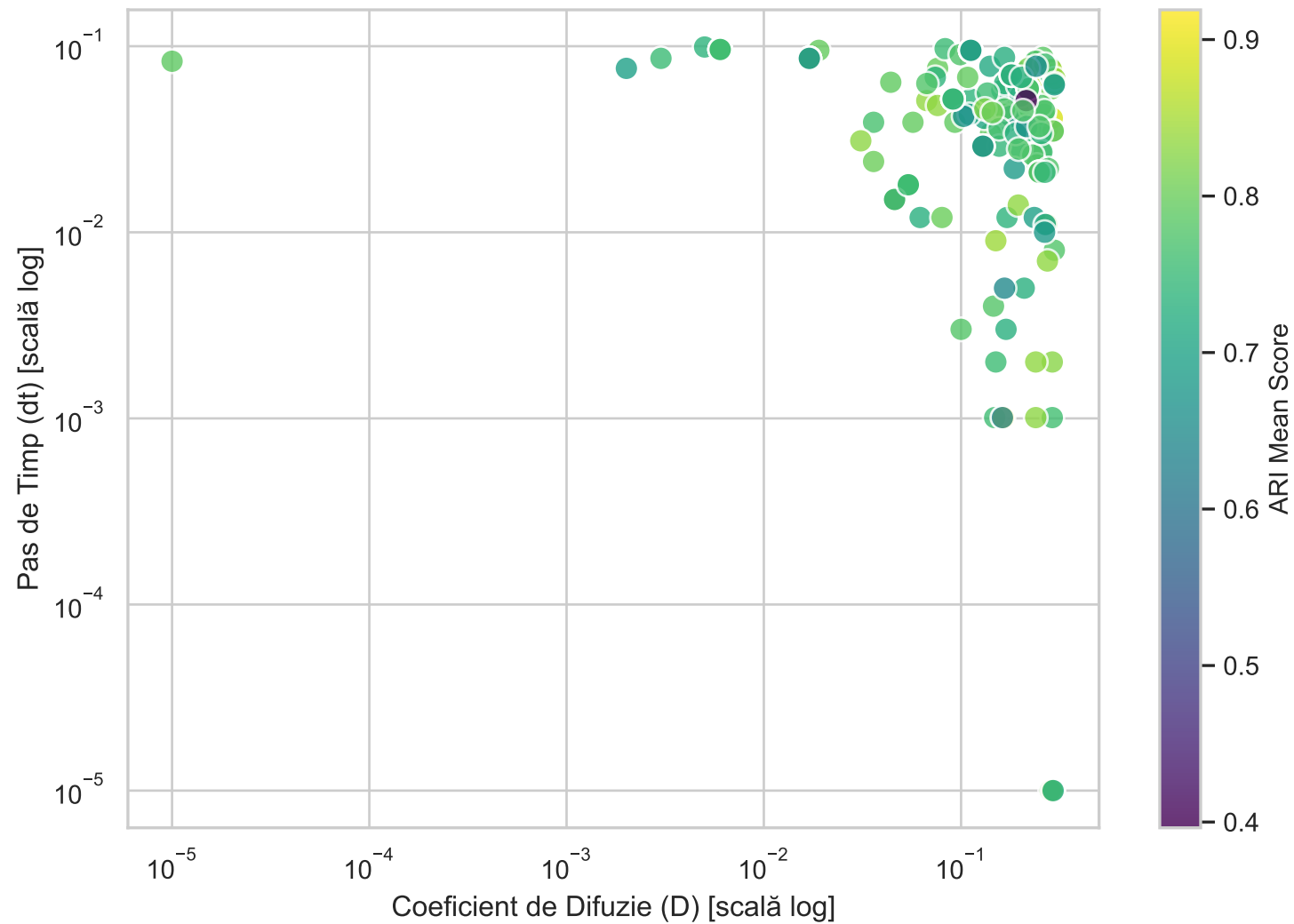
ARI Mean în funcție de D și dt
