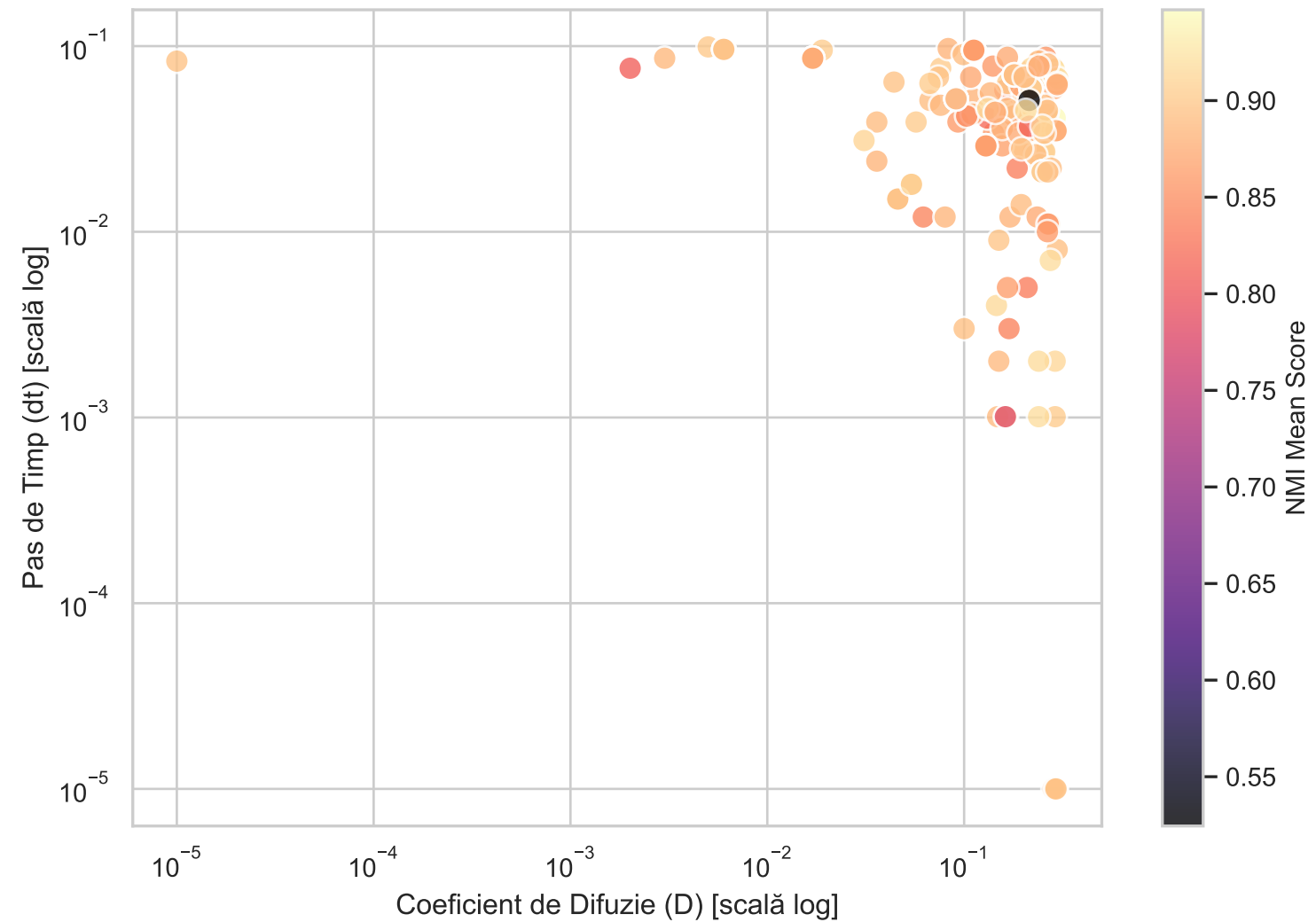
NMI Mean în funcție de D și dt
